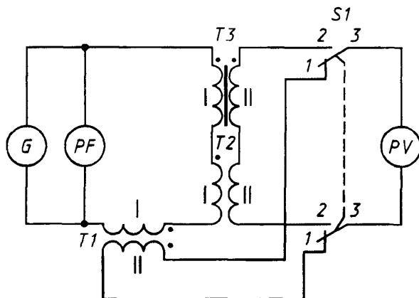
Рисунок 1 — Схема для измерений в динамическом режиме перематгничивания
