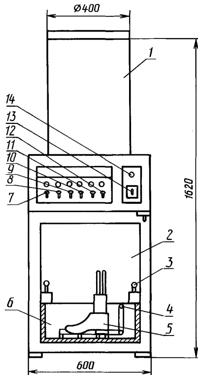
Прибор для определения пылепроницаемости спецобуви ЭПОП
