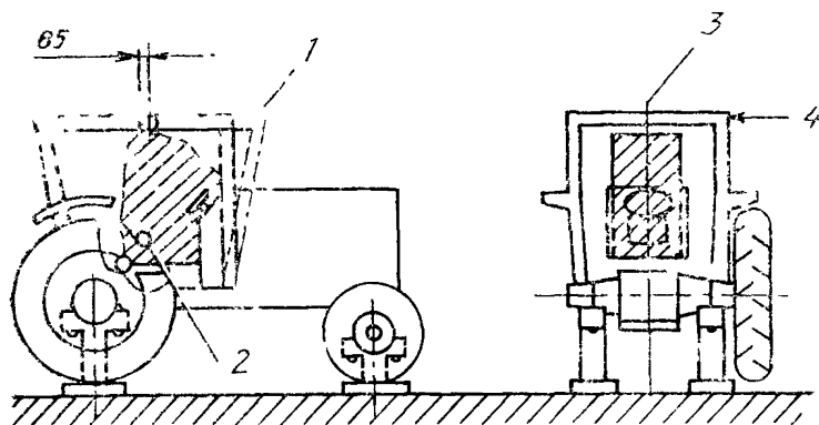
1 деформация под действием продольного нагружения сзади 2 — контрольная точка сиденья, 3 — продольная центральная линия проходящая через контрольную точку сиденья 4 — нагрузка
