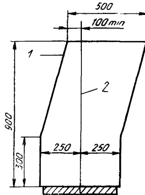
1 — нагрузка 2 — вертикальная основная плоскость
