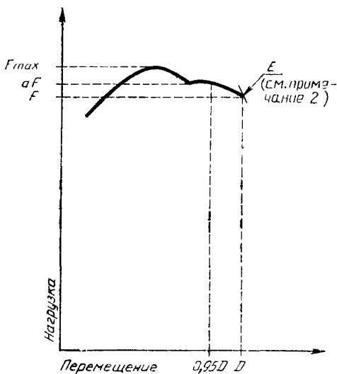
Диаграмма нагрузка — перемещение
