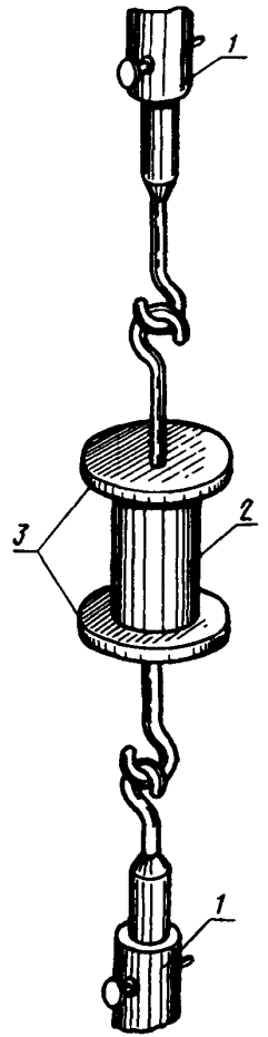
1 — зажим; 2 — образец; 3 — пластины
