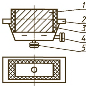
1 — образец; 2 — держатель; 3 — замазка; 4 — патрубок для подвода воздуха; 5 — патрубок для присоединения манометра
