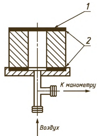
1 — промасленная калька или вакуумная резина; 2 — замазка
