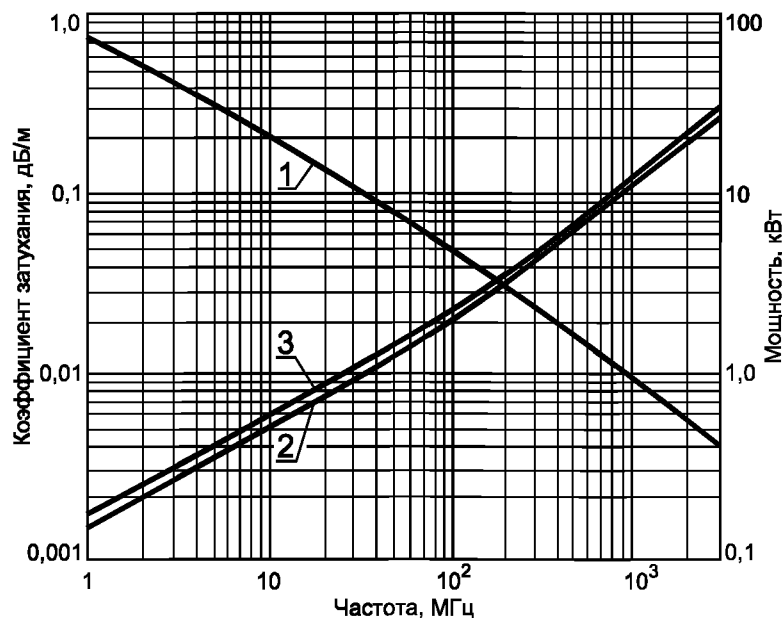
Частотные зависимости
