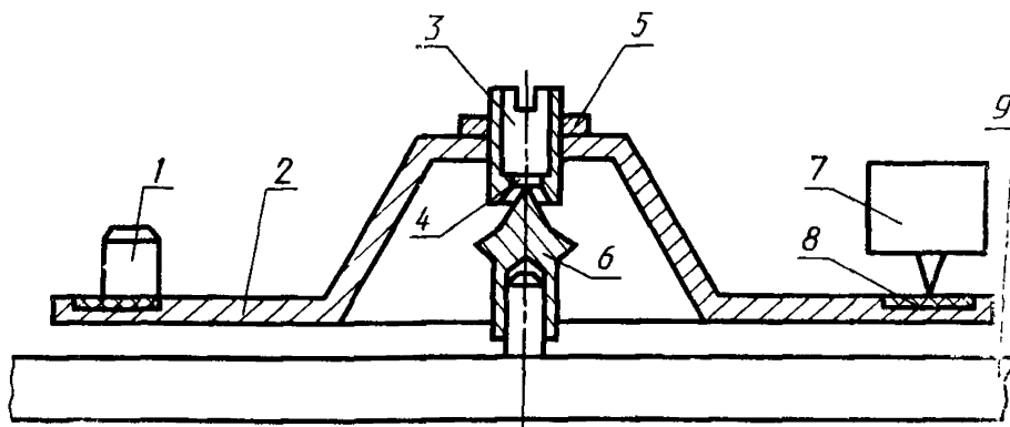
1 — противовес; 2 — диск; 3 — втулка; 4 — подпятник; 5 — стопорная гайка; 6 — опора; 7 — головка звукоснимателя; 8 — кольцо из материала грампластинки; 9 — диск ЭПУ
