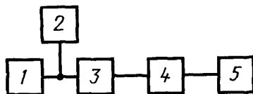
1—сеть и автотрансформатор (п. 4.2.11) или источник питания (п. 4.2.20); 2—вольтметр (п. 4.2.8); 3—ЭФ (ЭП, ЭПУ) с грампластинкой (п. 4.2.13); 4—прибор (п. 4.2.2); 5—электронно-счетный частотомер (п. 4.2.4)
