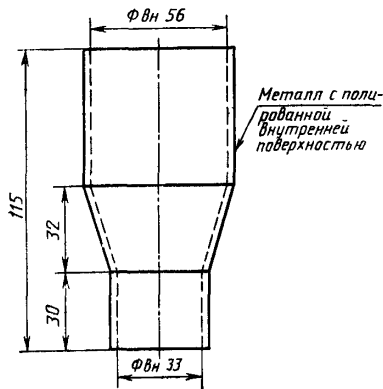
Воронка для определения насыпной плотности
