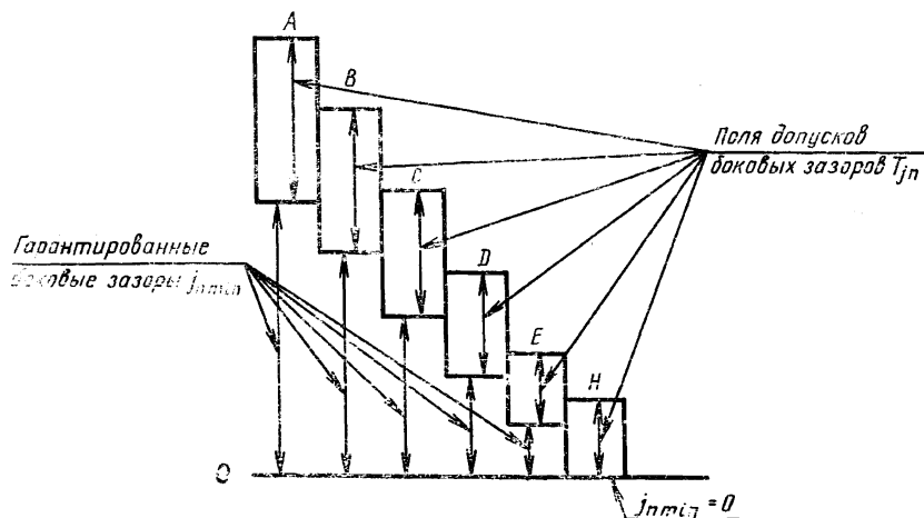
Виды сопряжений и гарантированные боковые зазоры
