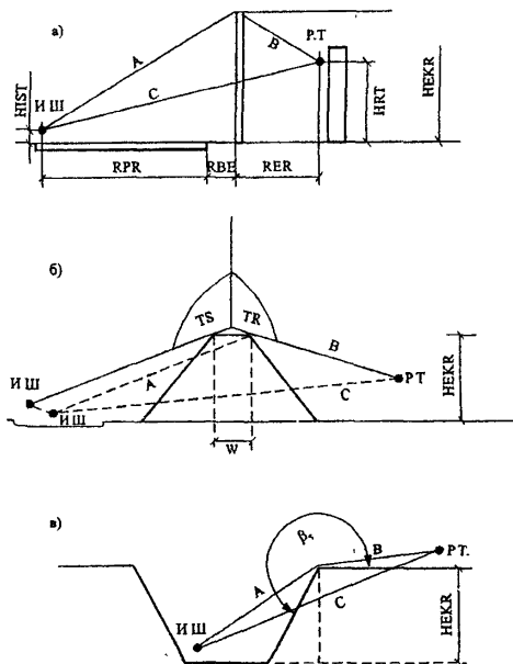
Рис. 4.12. Схема для расчета разности хода звуковых лучей в случае: а - экрана-сетки; б - экрана-насыти; в - экрана-выемки
