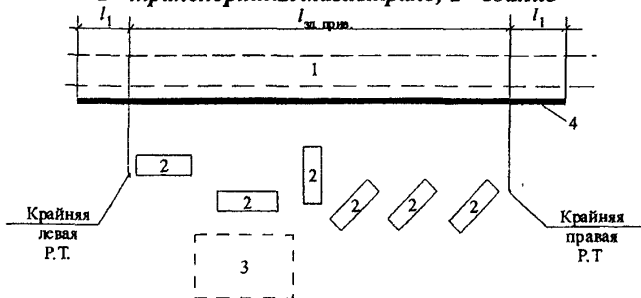
Рис. 4.6. Определение требуемой длины экрана для защиты от шума магистрали группы зданий: 1 - транспортная магистраль; 2 - здания; 3 - площадка отдыха; 4 - экран; • - расчетная точка
