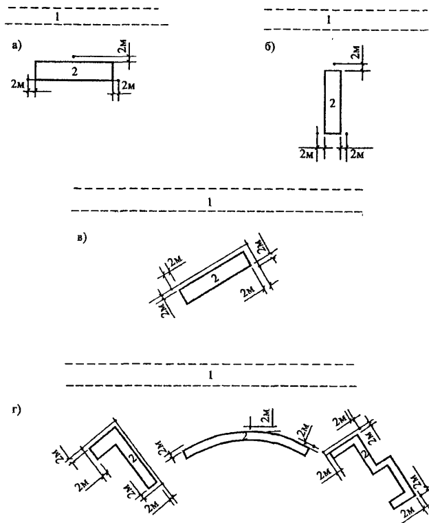
Рис. 4.3. Выбор расчетных точек около здания: а - фронтальное расположение; б - торцевое расположение в - расположение под углом к магистрали; г - здание сложной формы; 1 - транспортная магистраль; 2 - здания; • - расчетные точки
