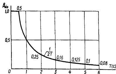
Рис.5. График нормированного коэффициента динамичности вектора углового ускорения вращения сейсмического воздействия \bar{\beta}_{\ddot{\alpha}_0}(\Gamma)
