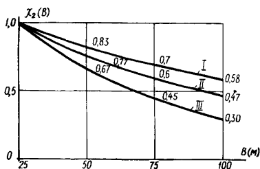
Рис.3. Графики нормированных функций \chi_2(B) = e^{\delta(B-25)} при \delta = -7,2 \cdot 10^{-3} ; -1 \cdot 10^{-2} и -1,6 \cdot 10^{-2} (1/м) для I, II и III категорий грунтов, соответственно.
