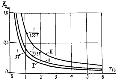
Рис. 4. Графики нормированных коэффициентов динамичности вектора ускорения поступательного движения сейсмического воздействия \bar{\beta}_{\ddot{x}_0}(\tau) для грунтов I, II и III категорий
