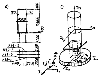
Рис.6. Конструктивная схема (а) и расчетная динамическая модель (б) силосного корпуса
