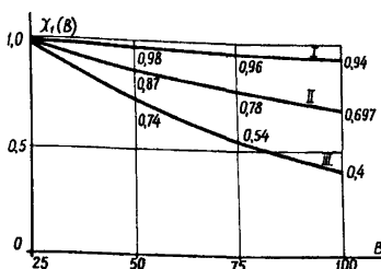
Рис.2. Графики нормированных функций \chi_1(B) = e^{\alpha(B-25)} при \alpha = -8 \cdot 10^{-4} ; -4,8 \cdot 10^{-3} и -1,2 \cdot 10^{-2} (1/м) для I, II и III категорий грунтов, соответственно
