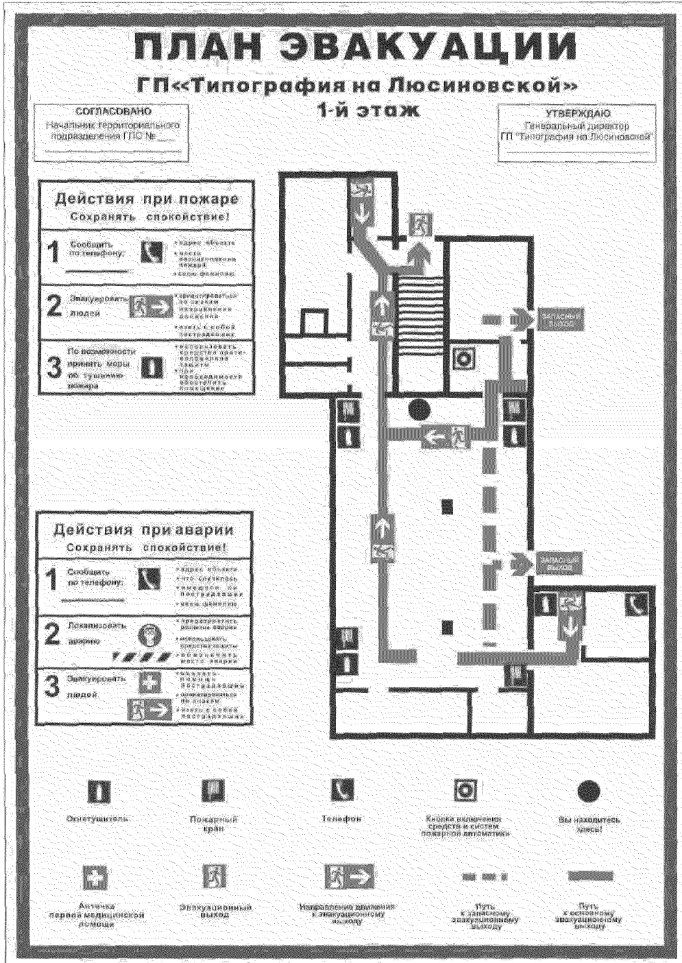
Рисунок В.1 – Этажный план эвакуации (фотолуминесцентный)
