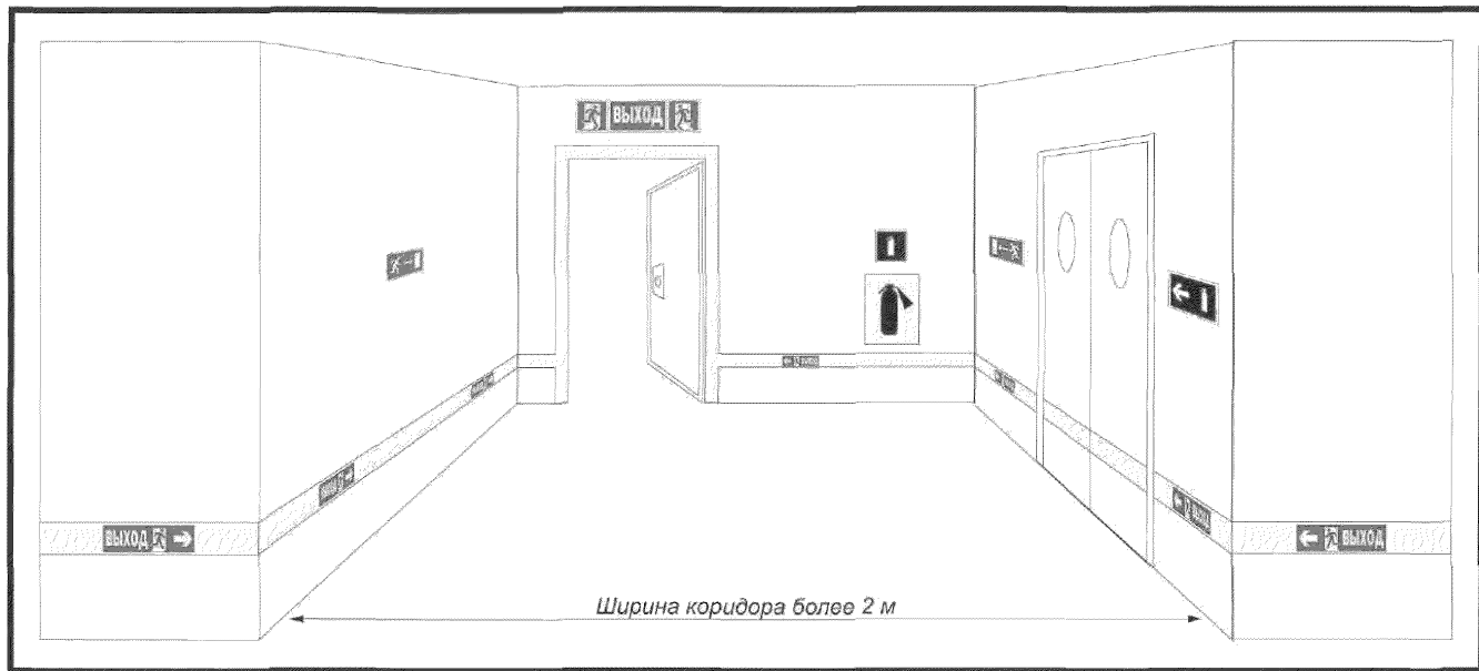
Рисунок Б.2 – Пример обозначения элементами ФЭС коридора. Направляющая полоса на правой стене переходит на поверхность полотна двери, не ведущей к выходу
