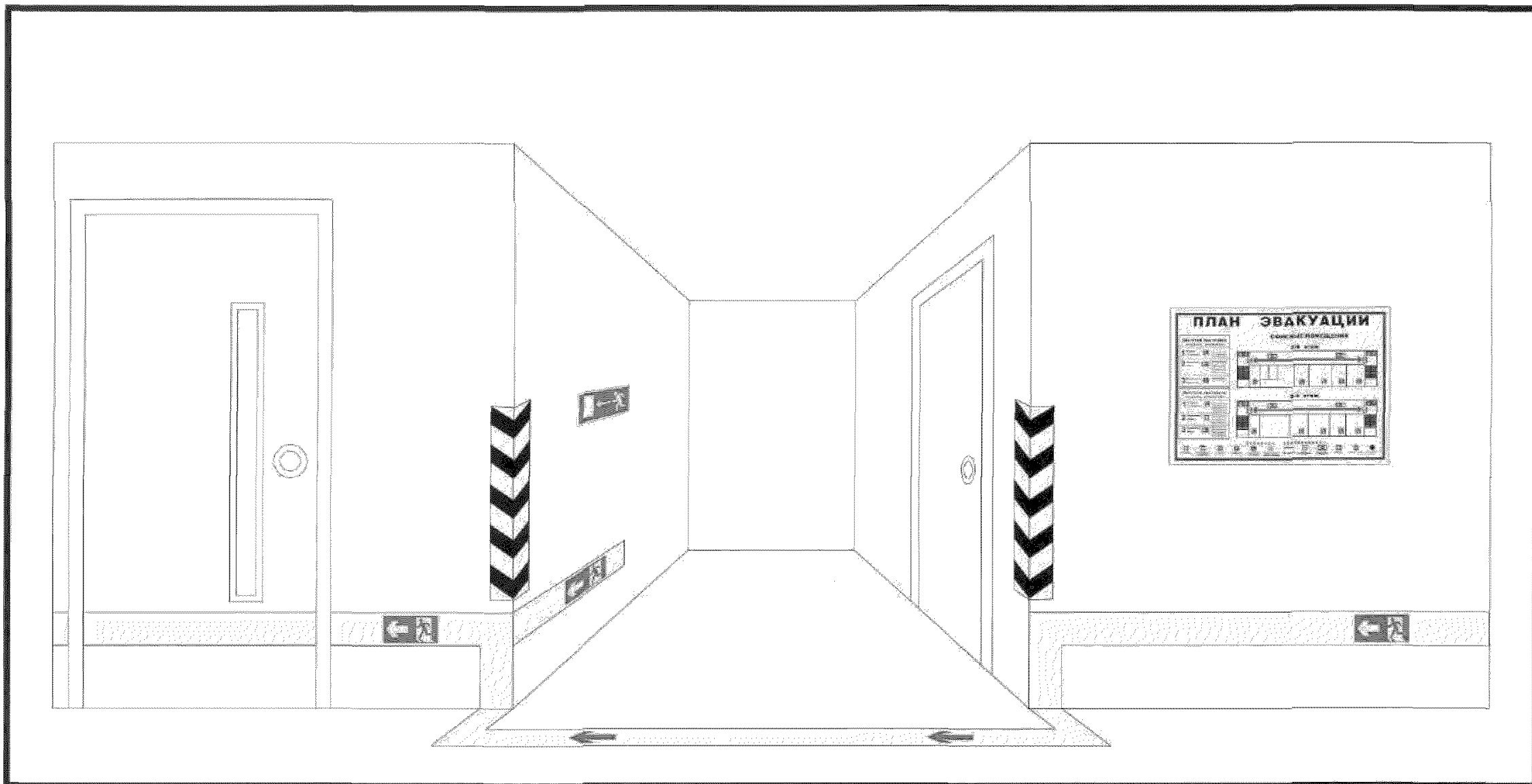
Рисунок Б.4 – Пример обозначения элементами ФЭС коридора при наличии тупика. Направляющая полоса переходит со стены на пол, исключая возможные разрыв в обозначении пути эвакуации, а затем снова переходит на стену
