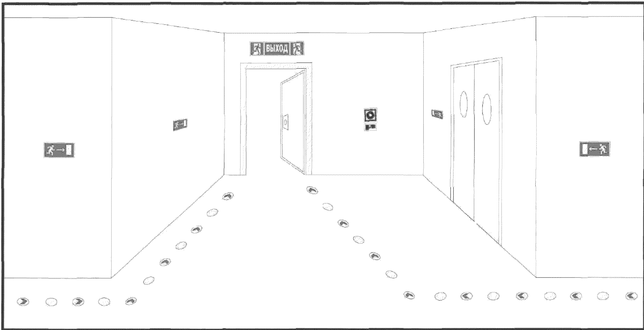
Рисунок Б.6 – Пример обозначения коридора элементами ФЭС с точечными (дискретными) направляющими линиями на полу, указывающими путь эвакуации
