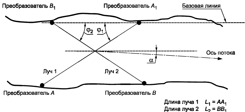
Рисунок 1 — Схема расположения преобразователей с пересекающимися лучами
