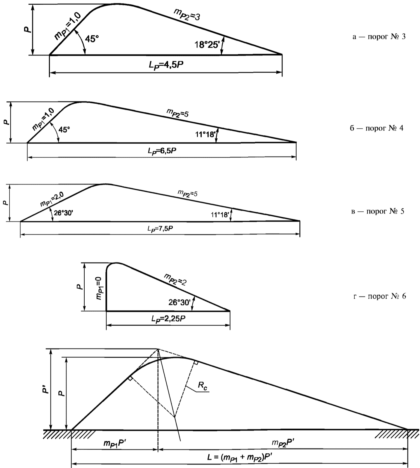
д — обозначения размеров продольного профиля порога
