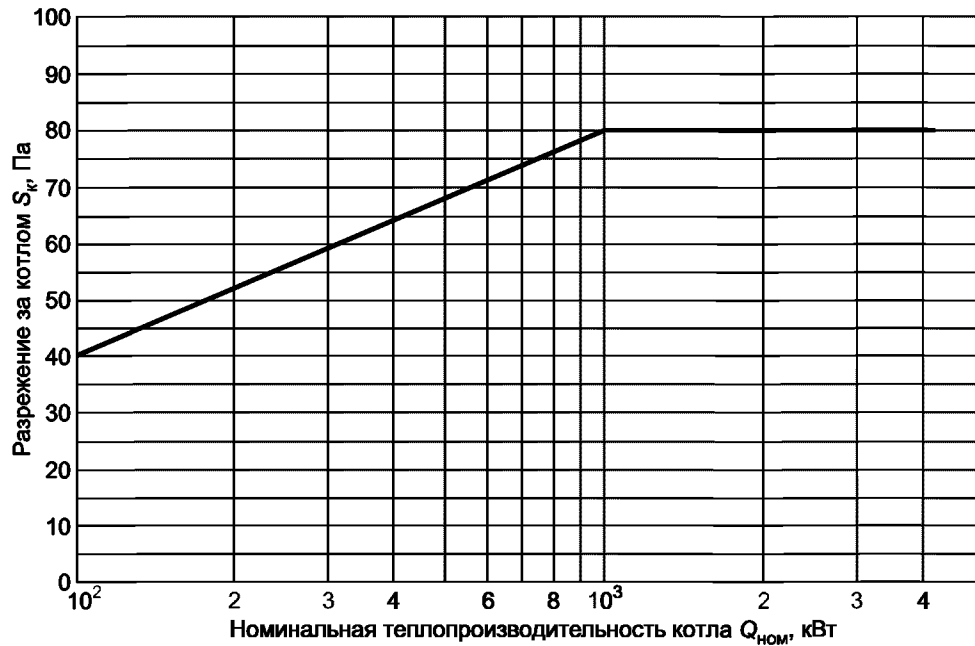
Рисунок 2 — Максимальное разрежение за котлом на естественной тяге
