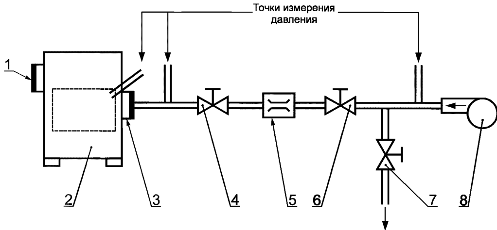
1 — патрубок уходящих газов; 2 — испытуемый котел; 3 — амбразура горелки; 4 — регулирующий орган 1; 5 — измеритель расхода; 6 — регулирующий орган 2; 7 — регулирующий орган 3; 8 — вентилятор
