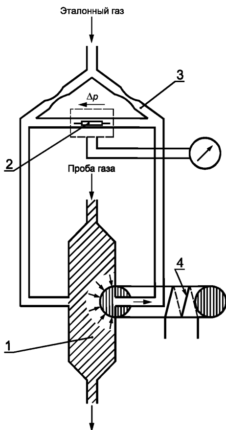
Рисунок 2 — Схема измерения концентрации NH 3
