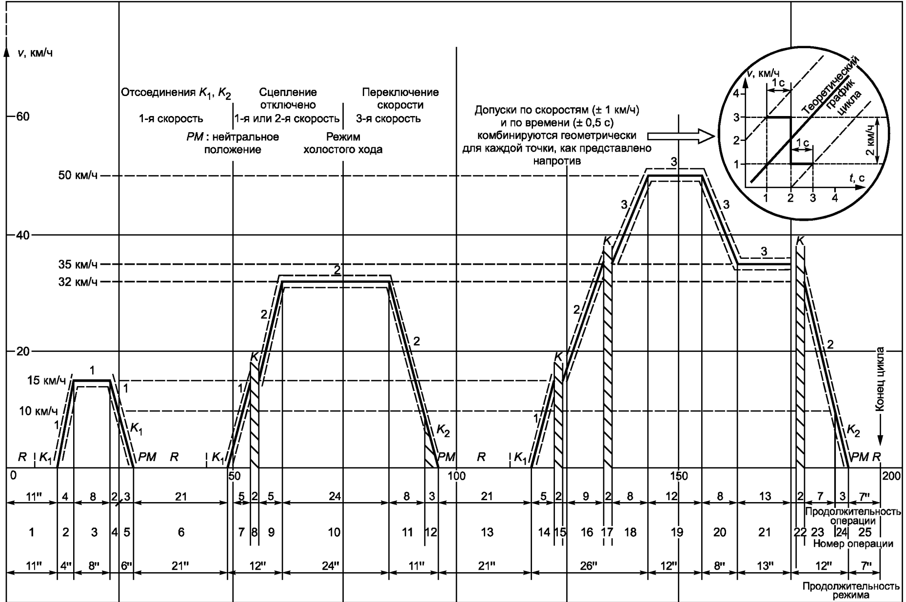
Рисунок 5.1 — Цикл движения для испытаний типа I
