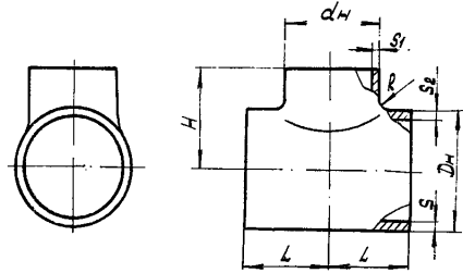
Тройник переходный
