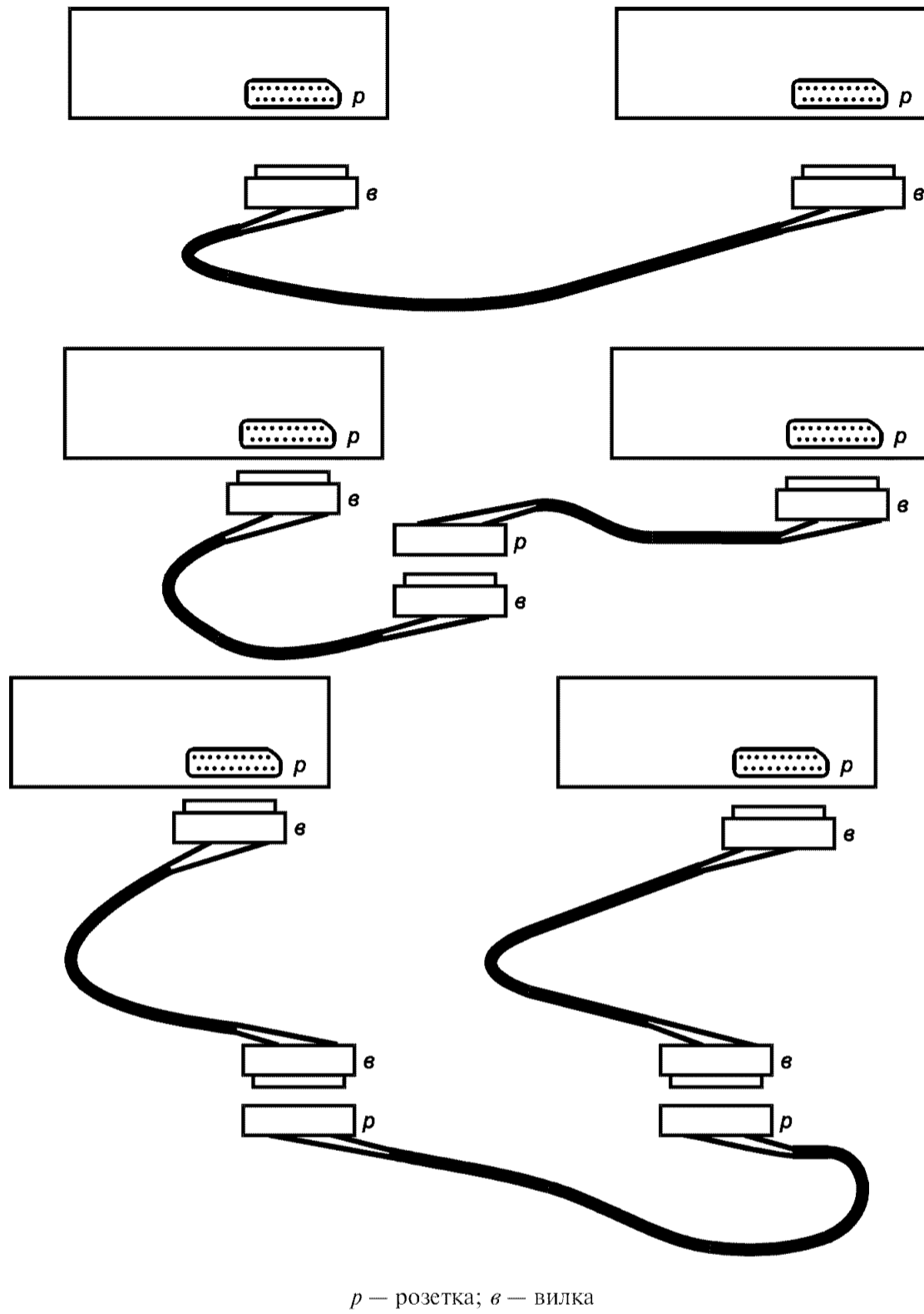
Рисунок В.2 — Виды соединительных шнуров
