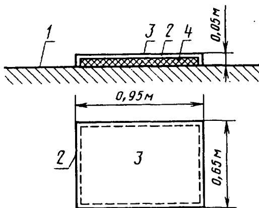
1 — стена; 2 — деревянная рама; 3 — фанера; 4 — стекловата или минераловата
