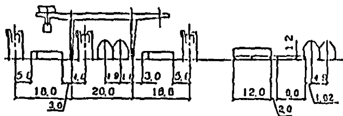
Рисунок 8.4 — Схема механизации №1 с портальными погрузчиками и размещением контейнеров параллельно линии кордона. Разрез
