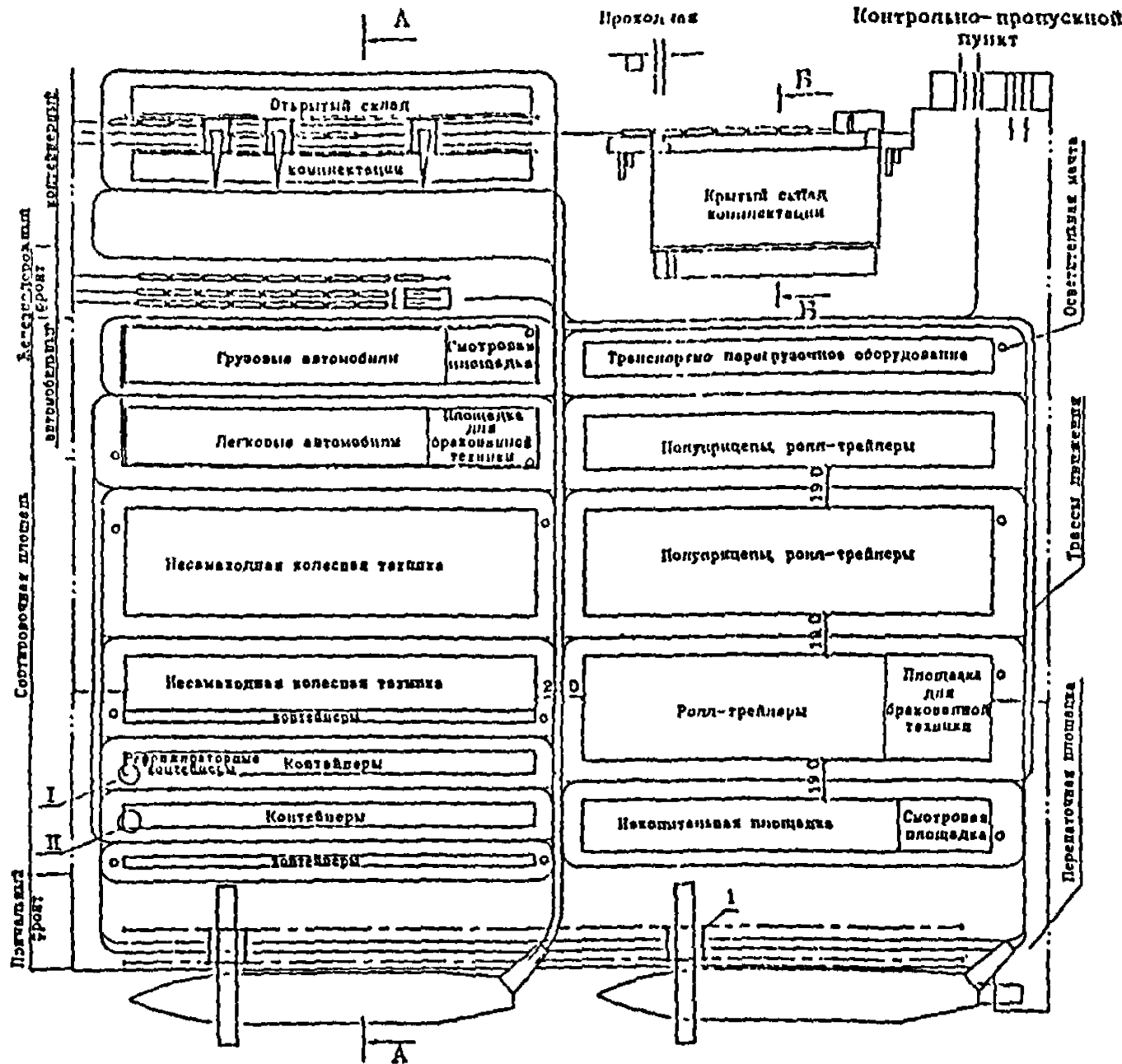
Рисунок 9.3 — Схема механизации N2 с использованием фронтальных погрузчиков. План.
