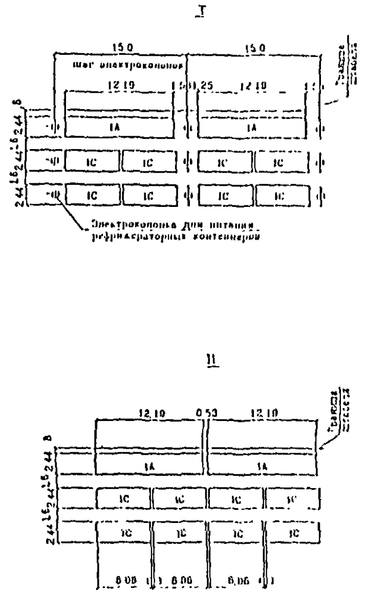
Рисунок 9.3 — Схема механизации И1 с портальными погрузчиками и размещением контейнеров параллельно линиям кордона (Витк)
