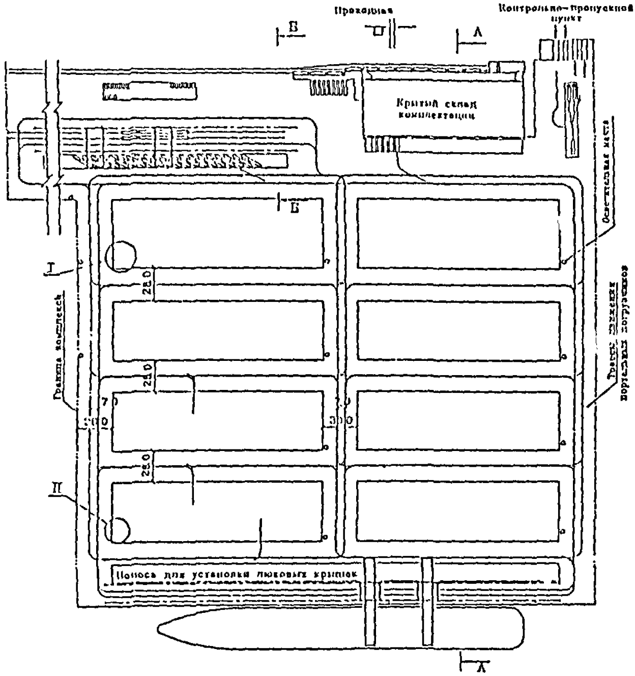
Рисунок 3.1 — Схема механизации №1 с портальными погрузчиками и размещением контейнеров партиями контейнерных машин корабля
