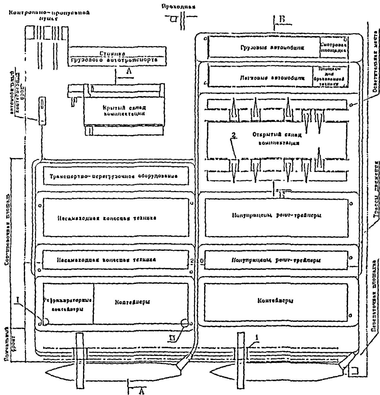
Рисунок 9.5 — Схема механизма №3 с использованием портальных погрузчиков.
