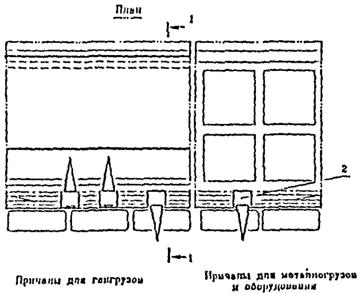
Рисунок 11.2 — Схема механизации Н2 разгрузки-выгрузки лихтеров портальными кранами
