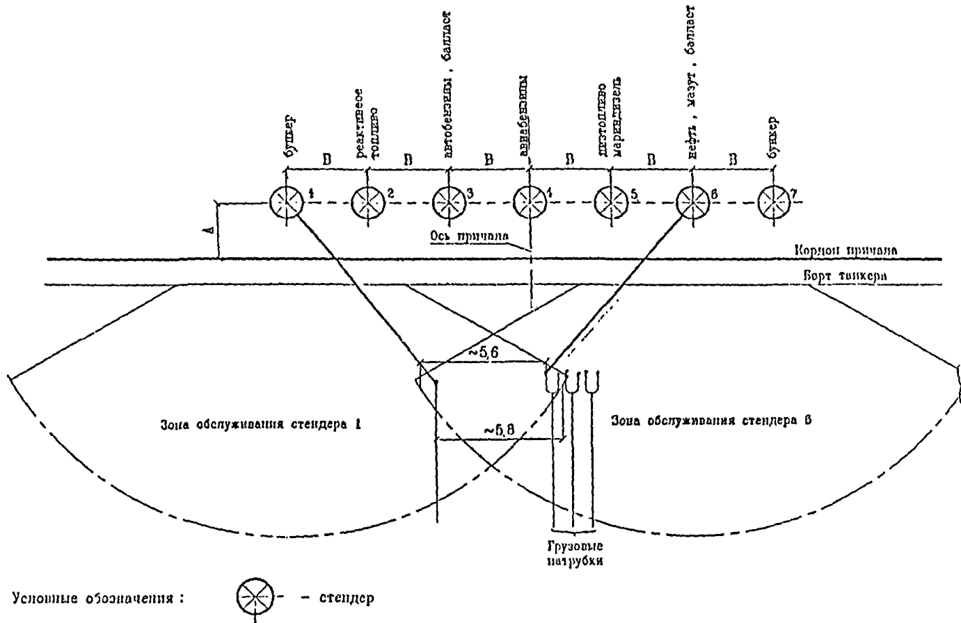
Рисунок 10.1 — Схема совмещения зон обслуживания стендеров с зоной расположения судовых пилонно-оперных
