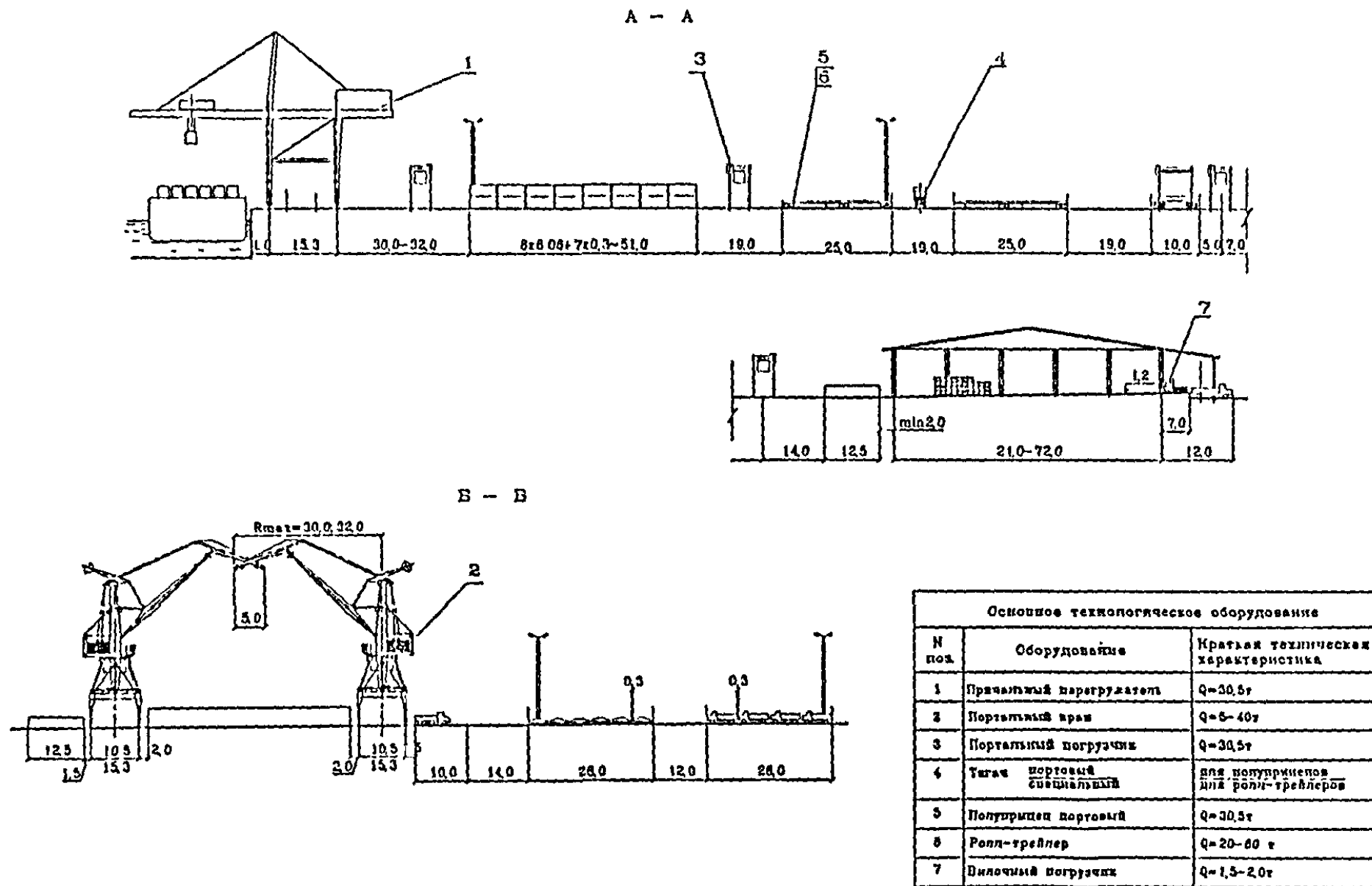
Рисунок 9.6 — Схема механизации №3 с использованием портальных погрузчиков. Разрезы
