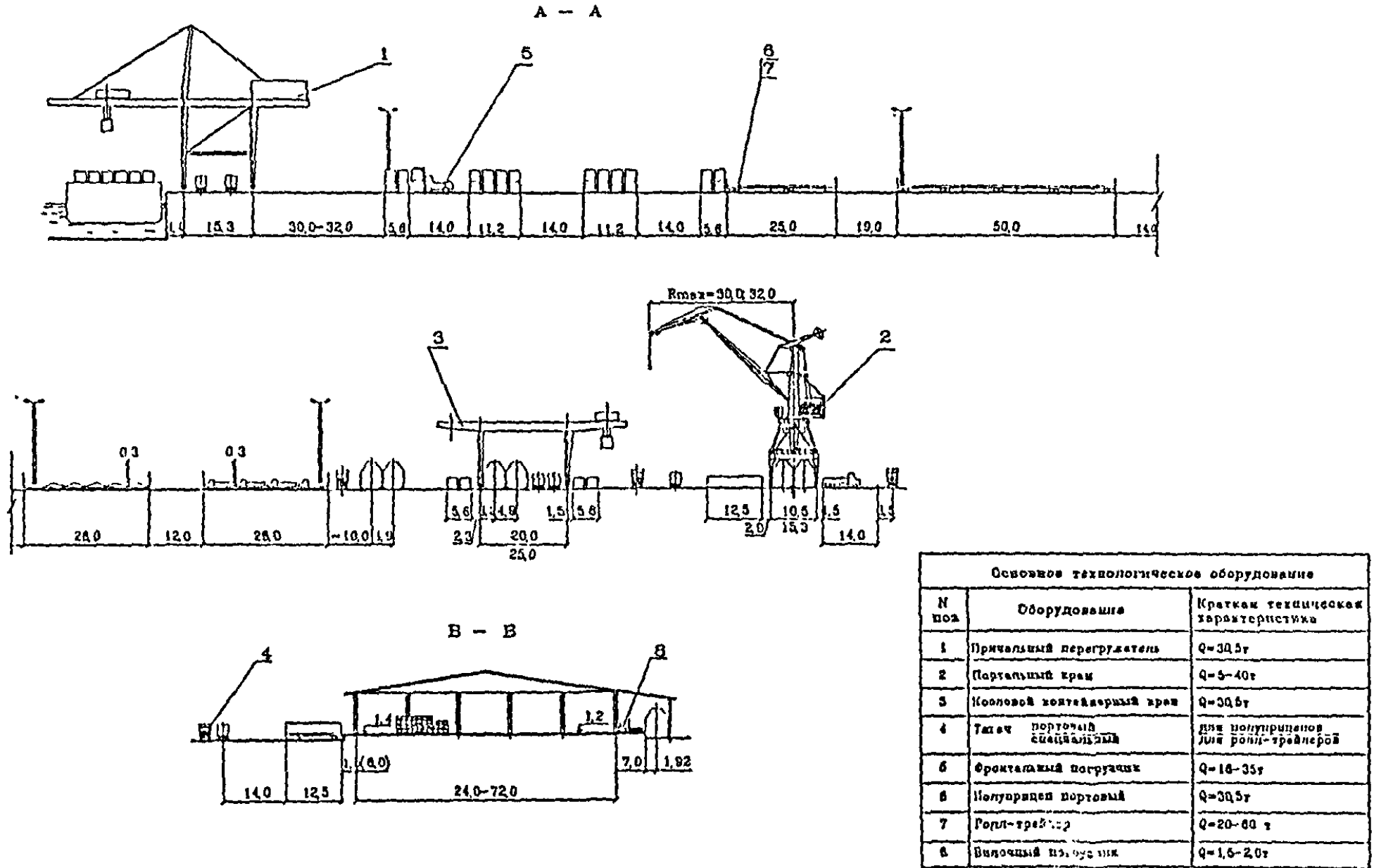
Рисунок 9.2 — Схема механизма N1 с использованием тягачей с полуприцепами. Разрезы
