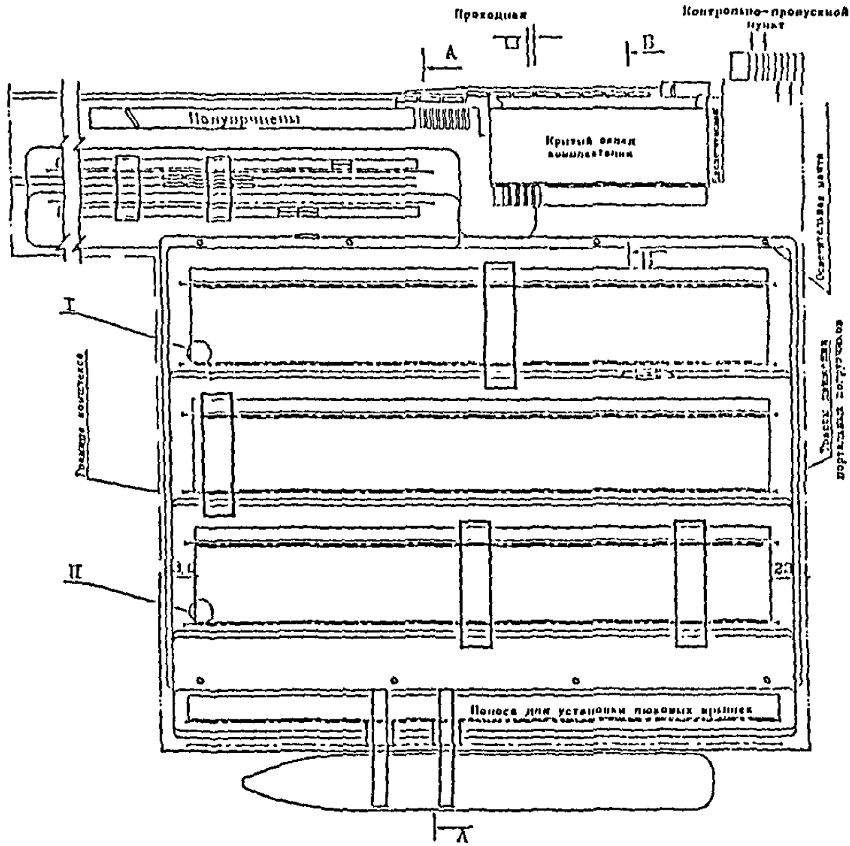
Рисунок 8.7 Схема механизации НЗ с коловыми перегружателями на рельсовом ходу II или
