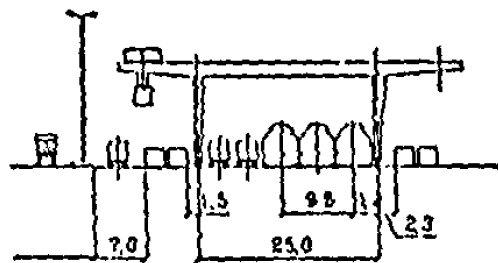
Вариант в 3-х железнодорожных путях на грузовой платформе
