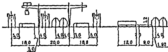
Вариант с 2х консольным козловым краном
