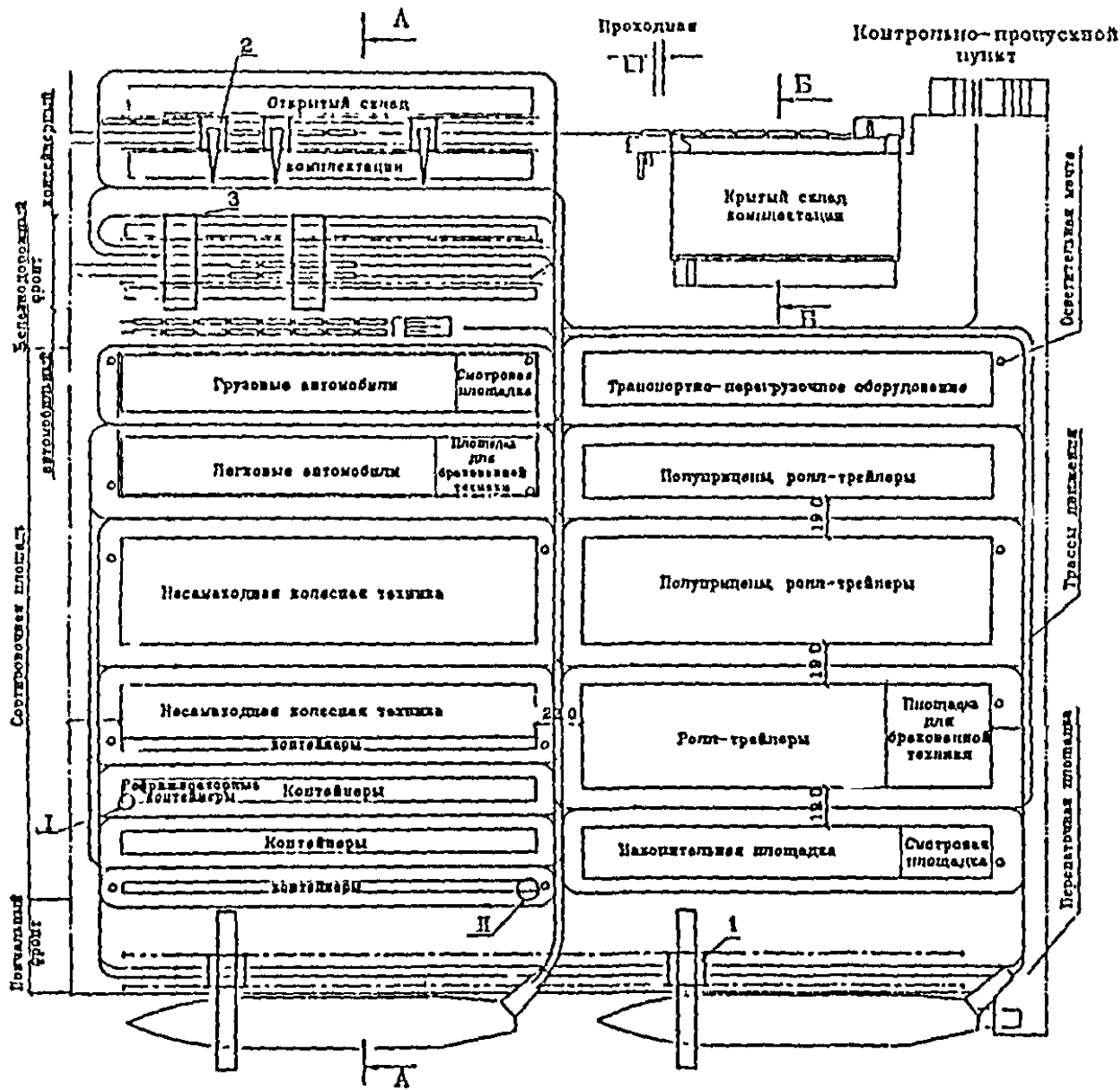
Рисунок 9.I — Схема механизации NI с использованием тягачей с полуприцепами Плак
