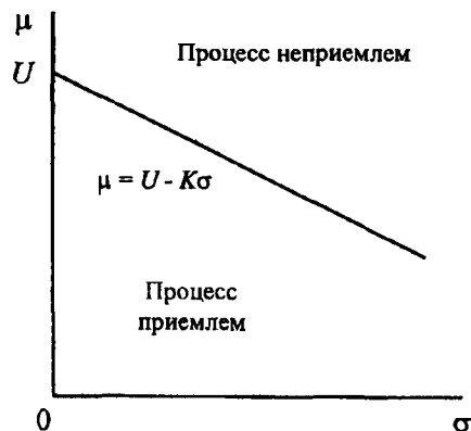
Рисунок 9 — Приемочная карта для верхнего предела поля допуска ( \sigma и \mu известны)
