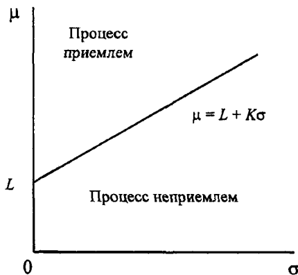
Рисунок 8 — Приемочная карта для нижнего предела поля допуска ( \sigma и \mu известны)
