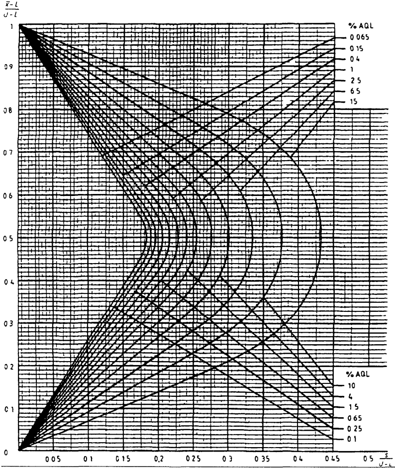
Диаграмма R-N — Кривые приемки для предельных значений с общим уровнем качества R-метод для кода объема выборки N (объем выборки — 20)
