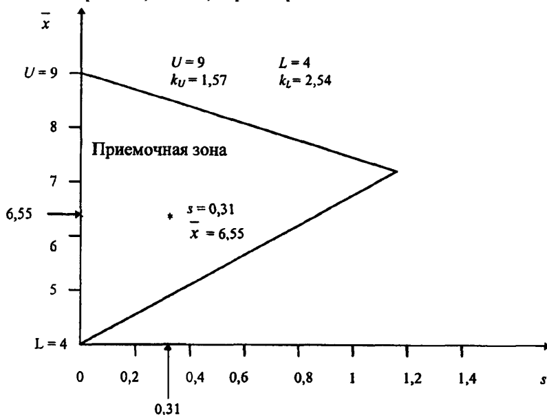
Рисунок 2 — Пример использования приемочной карты для двустороннего допуска (s-метод)
