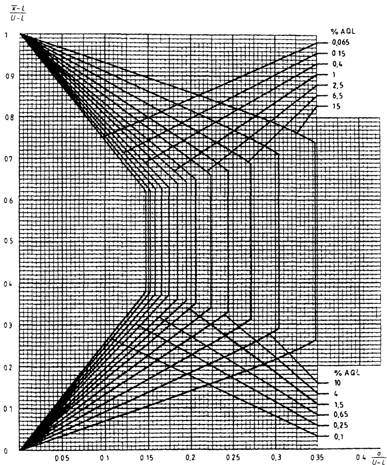
Диаграмма \sigma -I — Кривые приемки для предельных значений с общим уровнем качества. \sigma -метод для кода объема выборки J
