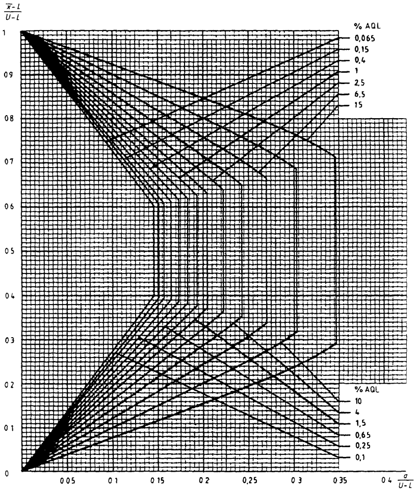
Диаграмма \sigma -К — Кривые приемки для предельных значений с общим уровнем качества. \sigma -метод для кода объема выборки К
