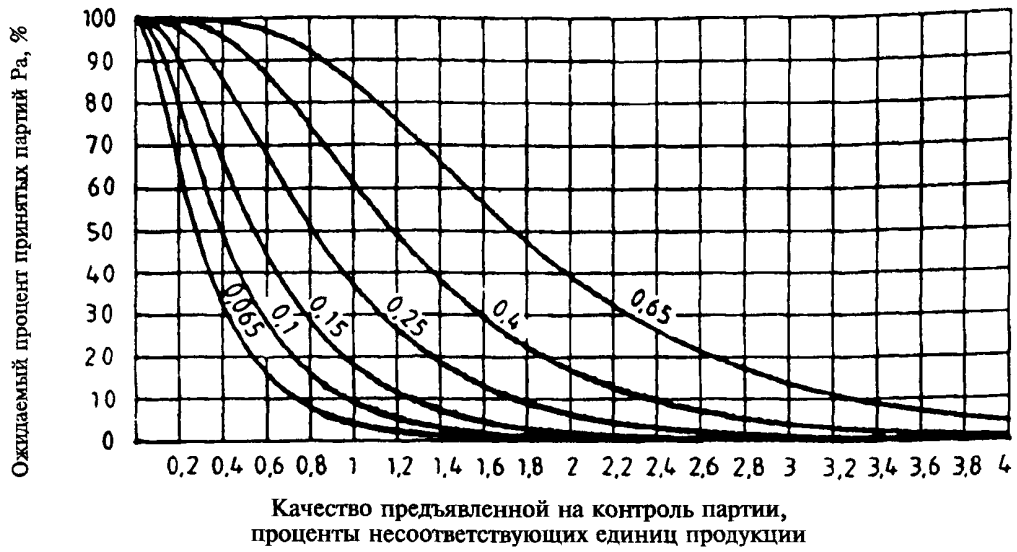
График VL — Оперативные характеристики для одноступенчатых выборочных планов контроля
