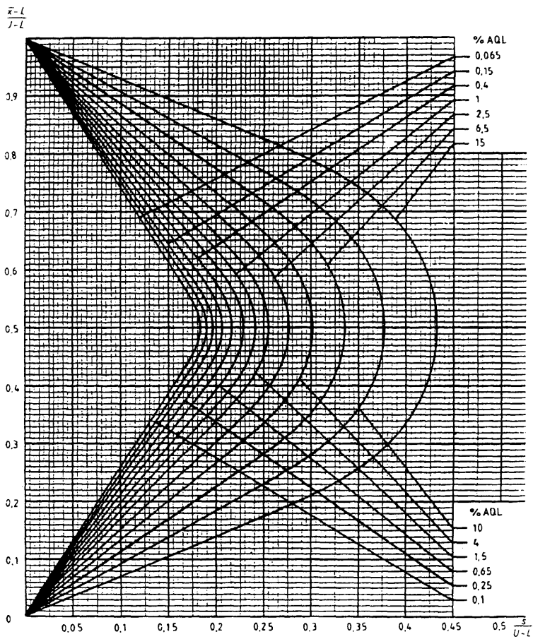
Диаграмма s-N — Кривые приемки для предельных значений с общим уровнем качества: s-метод для кода объема выборки N (объем выборки — 20)
