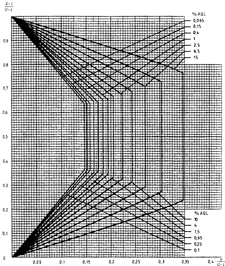
Диаграмма \sigma -G — Кривые приемки для предельных значений с общим уровнем качества: \sigma -метод для кода объема выборки G
