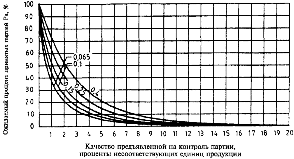
График VG — Оперативные характеристики для одноступенчатых выборочных планов контроля
