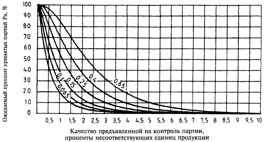
График VJ — Оперативные характеристики для одноступенчатых выборочных планов контроля
