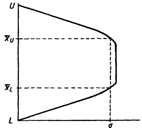
Рисунок 14 — Приемочная карта для предельных значений с общим уровнем качества
