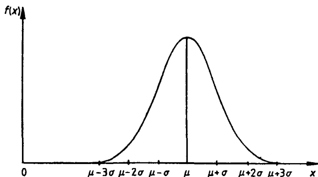
Рисунок 5 — Нормальное распределение
