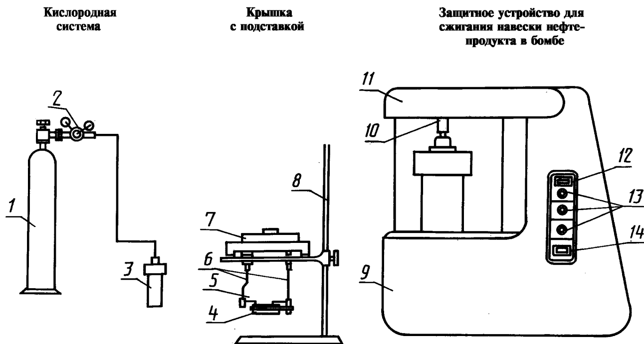
1 — баллон с кислородом; 2 — редуктор; 3 — калориметрическая бомба; 4 — тигель; 5 — запальная проволока; 6 — держатели тигля и запальной проволоки; 7 — крышка бомбы; 8 — подставка для крышки; 9 — корпус защитного устройства; 10 — клапан для сброса продуктов сгорания; 11 — крышка; 12 — кнопка «Сеть»; 13 — сигнальная лампа; 14 — кнопка «Запал»
