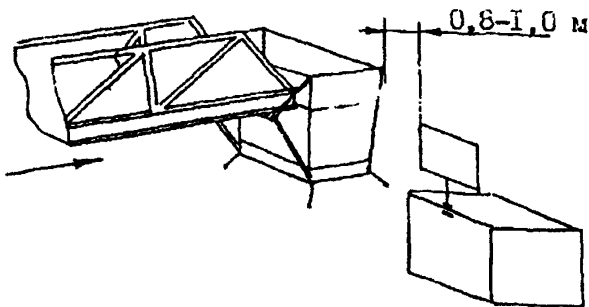
Рисунок 6.2. Движение вершины лестницы с люлькой за счет сдвига-выдвигания пакета колен
