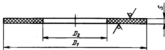
Размеры, мм
