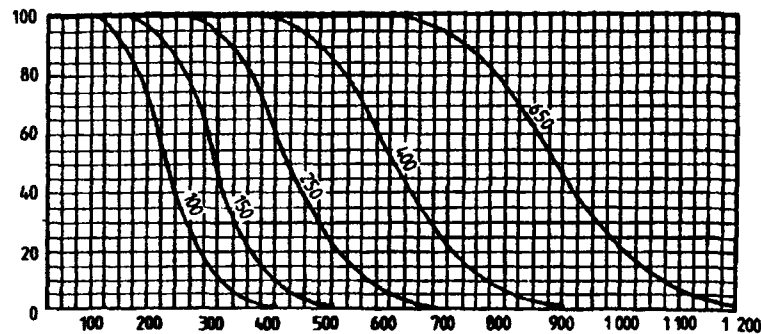
График С — Кривые оперативных характеристик для одноступенчатых планов (кривые двух- и многоступенчатого контроля по возможности максимально близки)
