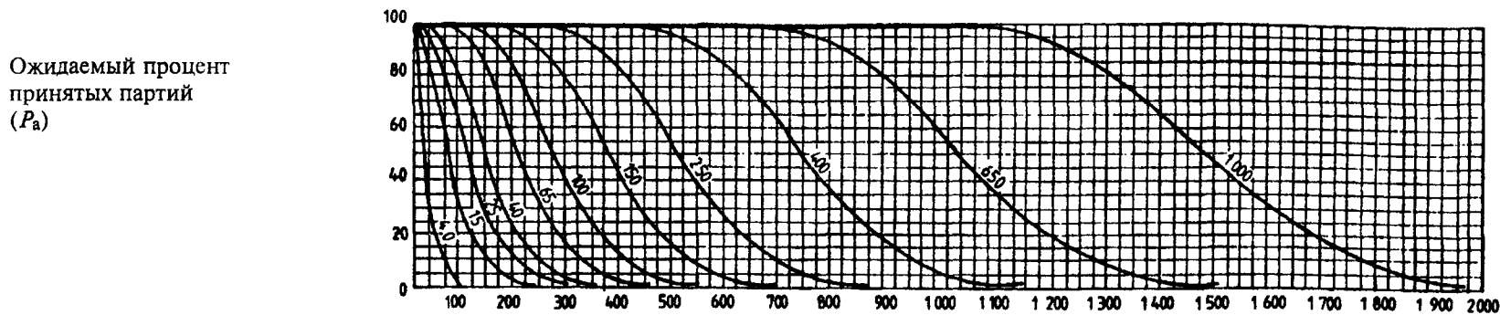
График А — Кривые оперативных характеристик для одноступенчатых планов (кривые двух- и многоступенчатого контроля по возможности максимально близки)
