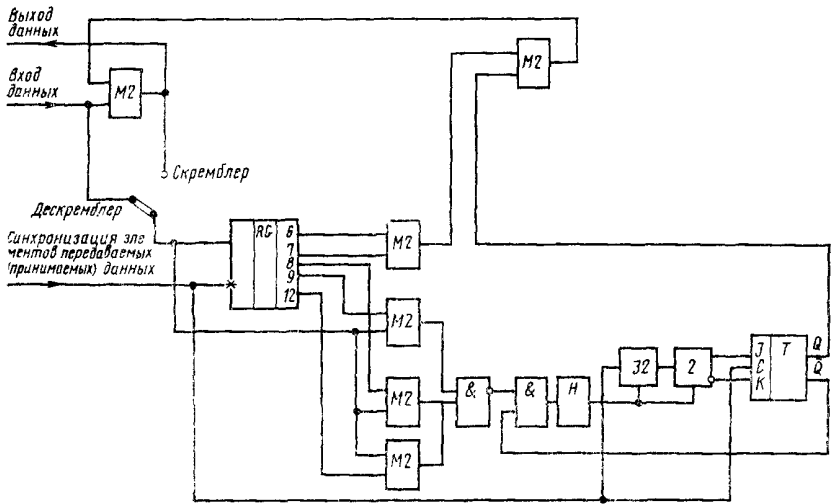
Функциональная схема скремблера-дескремблера для УПС-4,8 ТЧ
