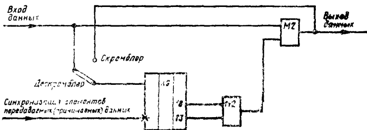
Функциональная схема скремблера-дескремблера для УПС-9,6 ТЧ
