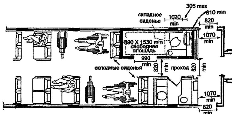
Б. Вагон с доступным туалетом
