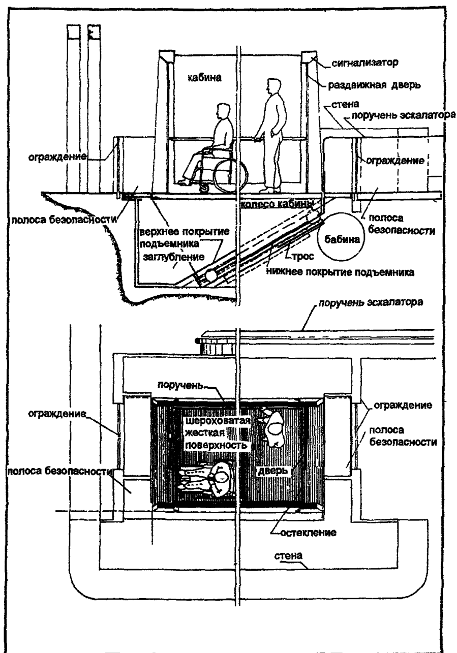
План и продольный разрез кабины (см. 7. 2.)
