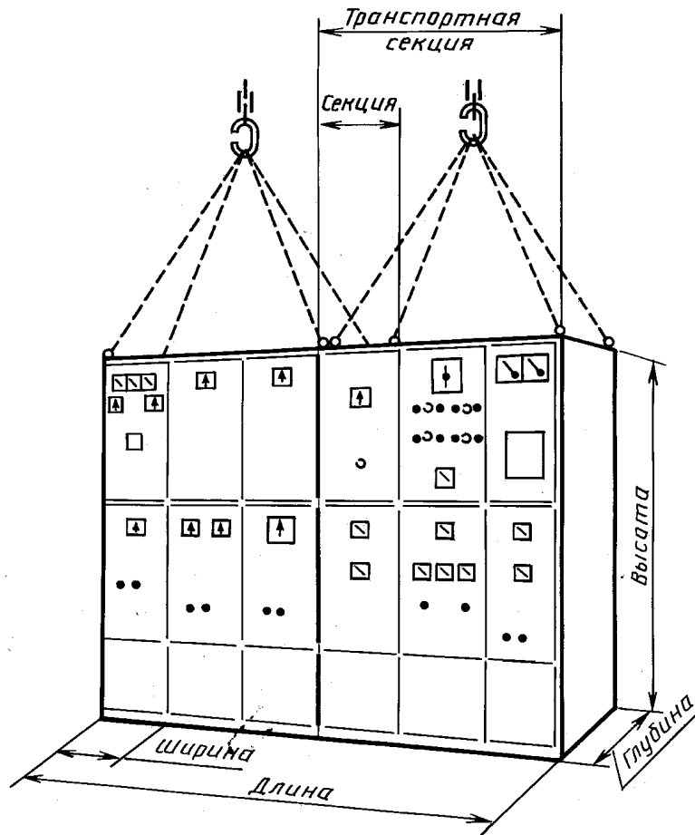
НКУ заводского изготовления многошкафного типа Черт. С.4
