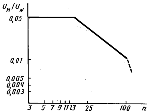
Максимально допустимая гармоническая составляющая номинального напряжения сети
