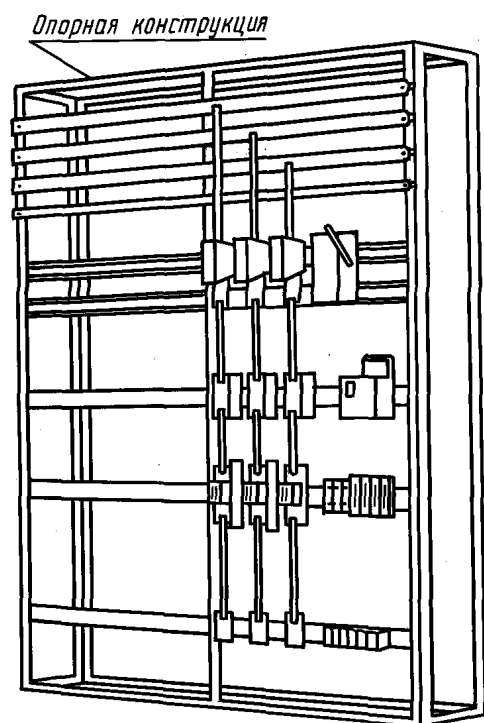
НКУ заводского изготовления открытого типа Черт. С.1
