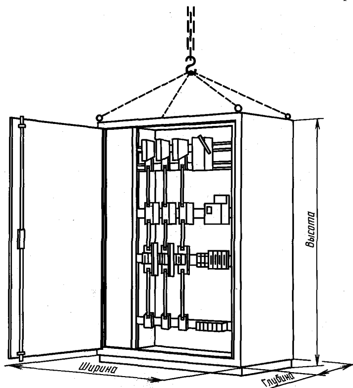
НКУ заводского изготовления шкафного типа Черт. С.3
