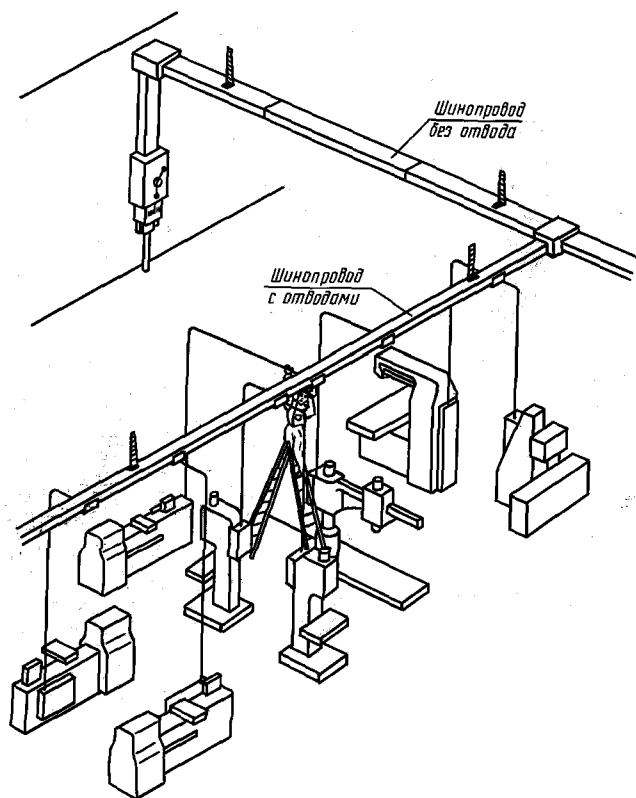
Система сборных шин (шинопровод)
