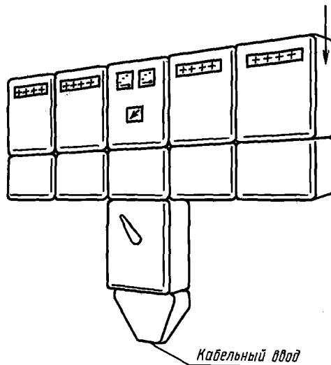
НКУ заводского изготовления многоящичного типа
