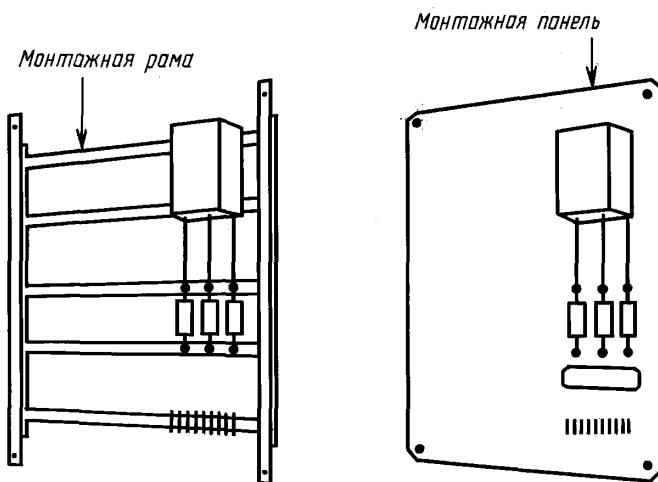
Неподвижные части
