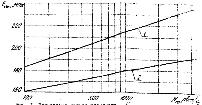
Рис. 1. Допустимые модули упругости E_{доп} одежды протире- совых автодорог, состоящие из одного (1) и из двух (2) слоев
