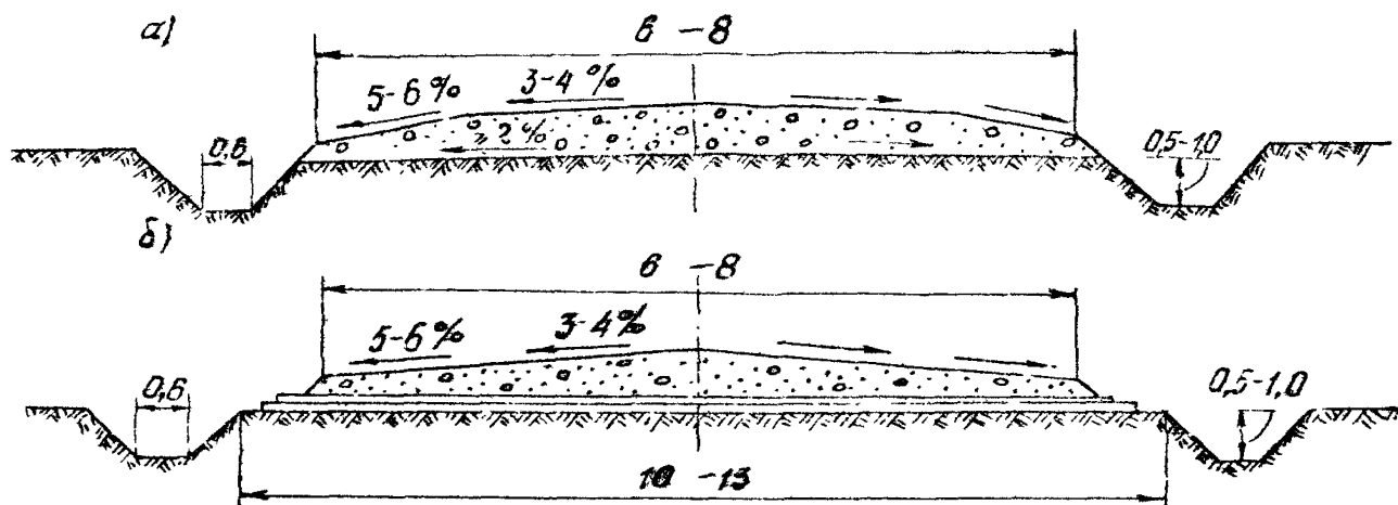
Рис. 7. Схемы насыпей в условиях I(а) и II(б) типов местности
