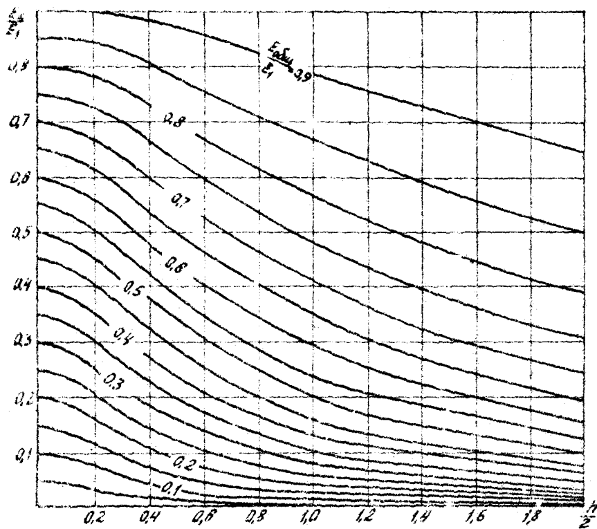
Рис. 2.номограмме для определения обшего модуля упругости двухосной системы
