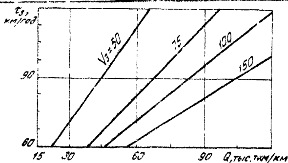
Рис. 1. График определения объема оперативных перевозок в рассматриваемом сечении дороги
