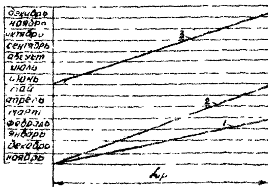
Рис. 2. График годового цикла этапного сооружения придорожной автомобильной дороги; 1, 2, 3 - этапы; L_k - Годовой прирост фронта строительства по трассе железной дороги
