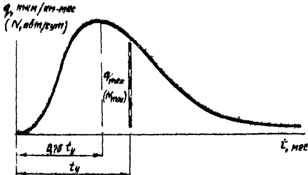
Рис. I. Кривая изменения грузонапряженности или интенсивности движения придорожной автомобильной дороги и ее основные параметры
