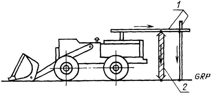
1—прямой стальной стержень; 2—стальная линейка
