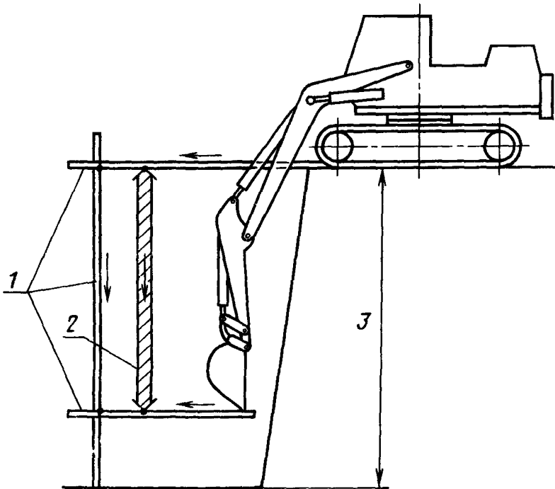
1—прямой стальной стержень; 2—стальная линейка; 3—высота
