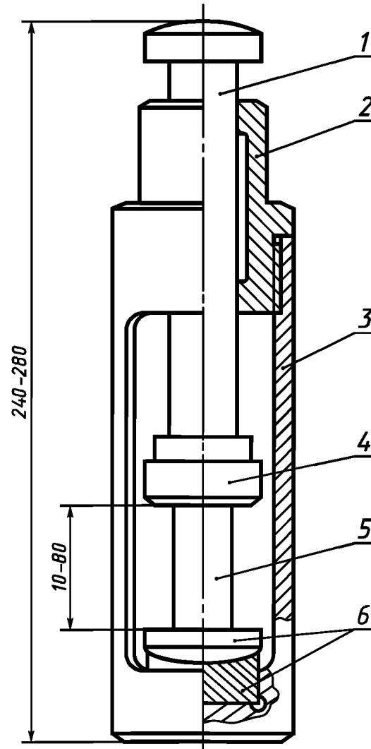
1 — пуансон; 2 — направляющая втулка; 3 — основание; 4 — опорная верхняя плита; 5 — образец; 6 — самоустанавливающая опора со сменным вкладышем
