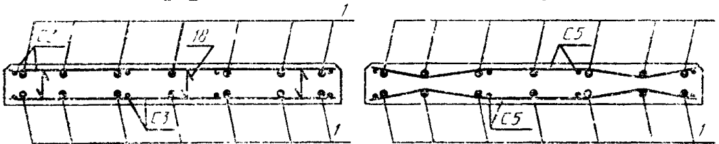
1 — напрягаемая арматура; 2 — крепление сеток С3
