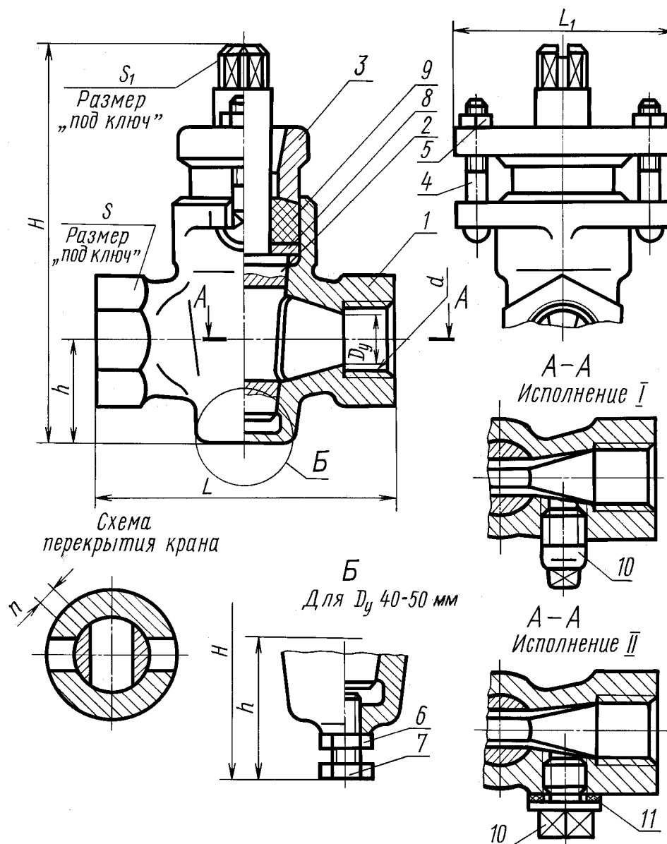
1 — корпус; 2 — пробка; 3 — втулка сальника фланцевая; 4 — болт анкерный; 5, 6 — гайки; 7 — болт; 8 — кольцо поднабивочное; 9 — набивка марки ПП; 10 — заглушка (пробка спускная); 11 — прокладка
