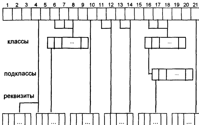
Рис. 2. Структура классификатора
