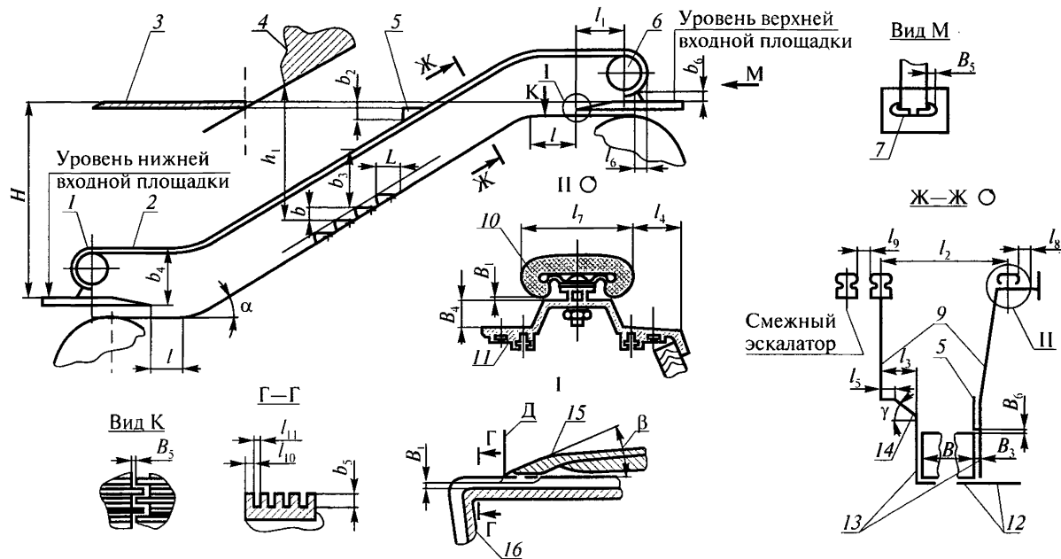
Рис. 1. Схема устройства эскалатора:
