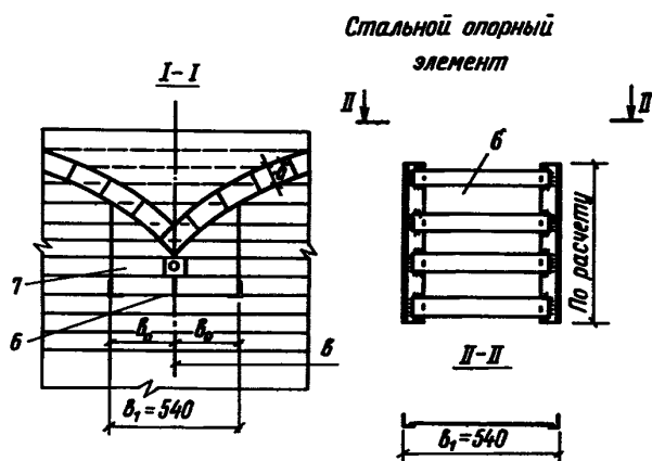
Черт. 72. Опорный узел свода двойной кривизны
