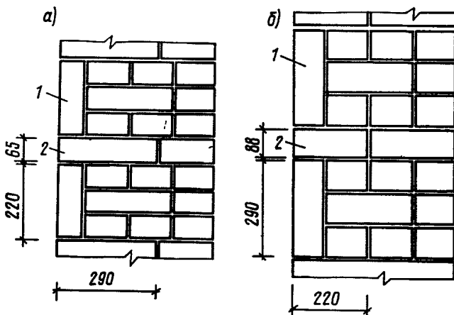
Черт. 46. Облицовка стен плоскими бетонными плитами a – из кирпича толщиной 65 мм; б – из кирпича толщиной 88 мм; 1 – плоские плиты; 2 – прокладной ряд из плит
