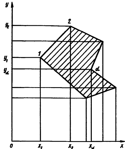
Черт. 1. Нумерация вершин горизонтальных сечений стен здания
