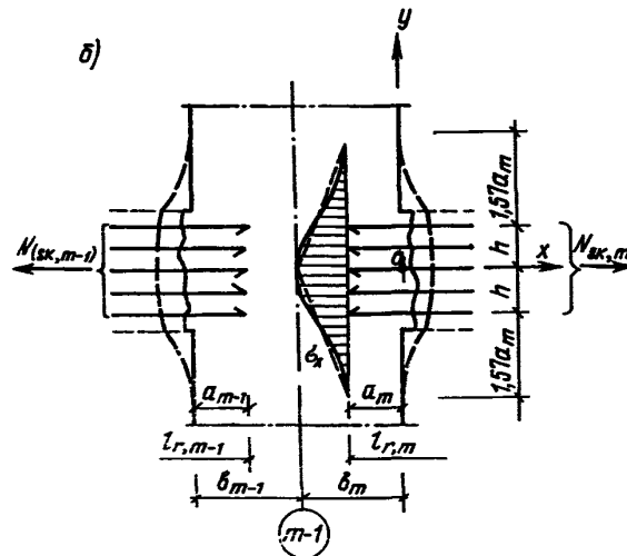
Черт. 8. Напряженно-деформированное состояние простенка в местах заделки в него элементов а — железобетонных или стальных; б — армированных
