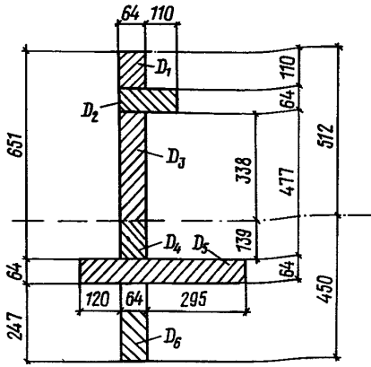
Черт. 22. Схема для определения коэффициента K стены № 1
