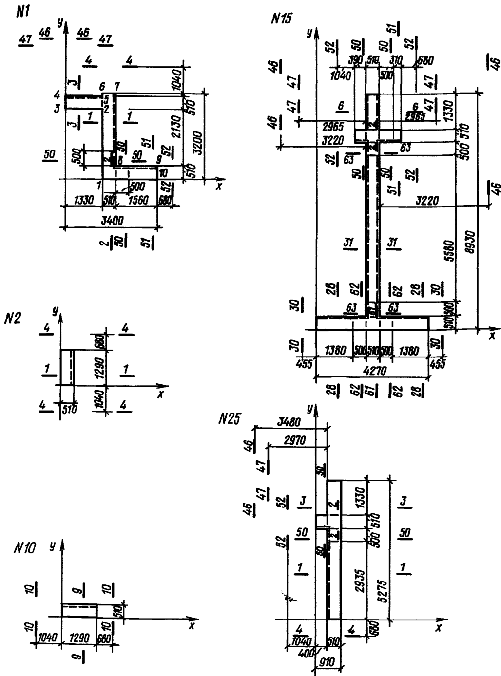
Черт. 11. Геометрические размеры горизонтальных сечений рассматриваемых элементов
