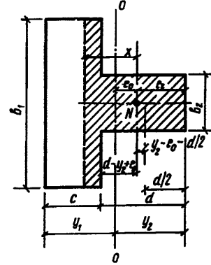
Черт. 1. Эксцентриситет в сторону полки
