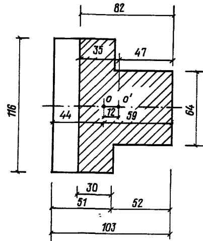
Черт. 6. Поперечное тавровое сечение
