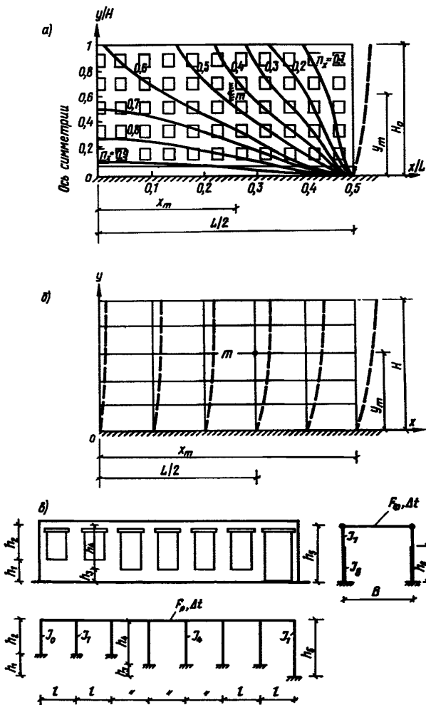
Черт. 6. Расчетные схемы каменных зданий
