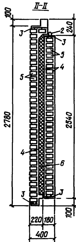
Черт. 34. Наружная стенная панель
