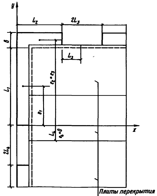
Черт. 5. Определение изгибающего момента от вертикальных нагрузок относительно оси Ox
