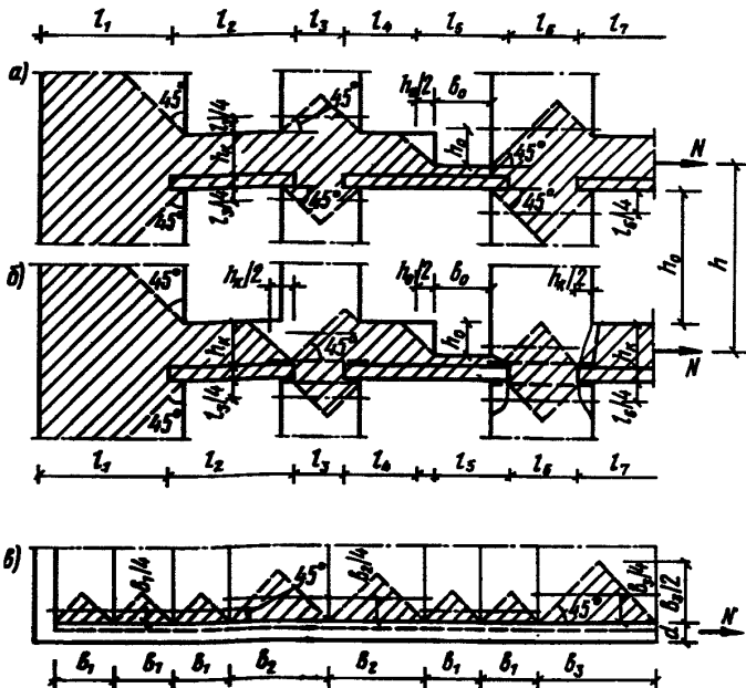
Черт. 3. Примеры построения зон влияния продольной силы N в кладке стен и перекрытий
