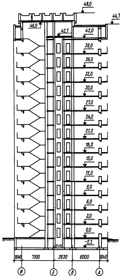
Черт. 9. Разрез здания
