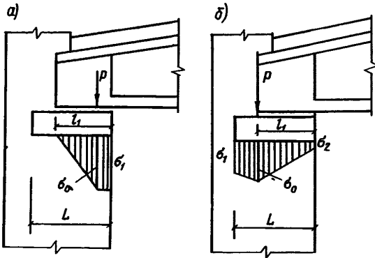
Черт. 4. Расчетная схема узла опирания балки на кладку
