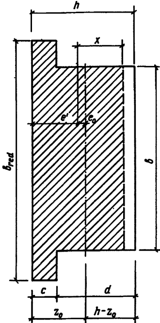
Черт. 49. Определение приведенной площади сечения про- стенка
