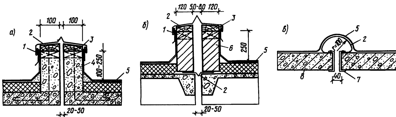
Черт. 62. Примеры устройства температурных швов в железобетонных крышах
