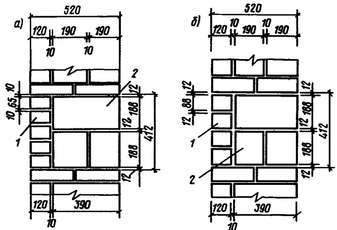
Черт. 47. Облицовка фасадов стен из бетонных камней a – с перевязкой прокладными тычковыми рядами кирпича толщиной 65 мм; б – то же, кирпич толщиной 88 мм; 1 – лицевой кирпич; 2 – бетонный камень
