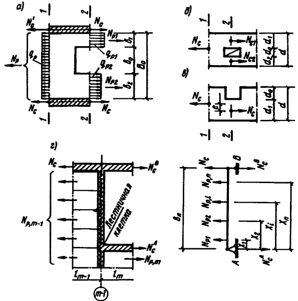
Черт. 7. К расчету продольных усилий в стенах и перекрытиях в местах ослабления отверстиями, штрабами и швами a — перекрытие с отверстием; b — кладка стены с отверстием; c — то же, со штрабой; d — лестничная клетка
