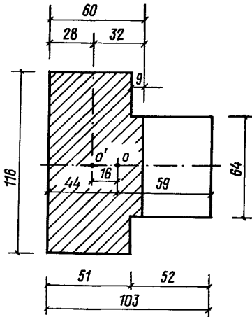
Черт. 7. Поперечное тавровое сечение
