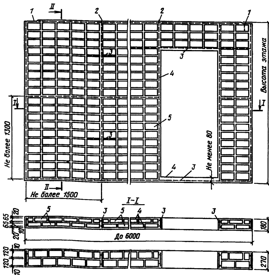
Черт. 35. Виброкирпичная перегородка
