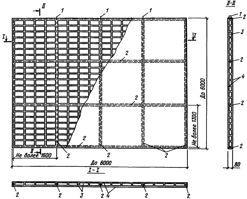
Черт. 36. Виброкирпичная перегородка 1 – монтажная петля; 2 – арматурный каркас; 3 – кирпич; 4 – растворный слой
