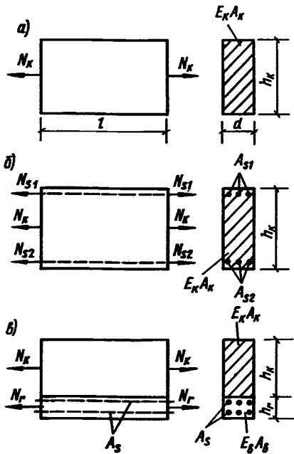
Черт. 2. Определение продольной жесткости неармированной и армированной кладки а — неармированная кладка; б — армированная кладка; в — кладка с железобетонным включением
