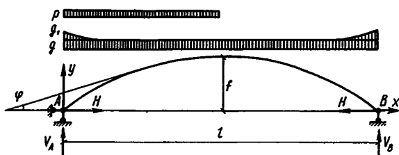
Черт. 70. Расчетная схема свода
