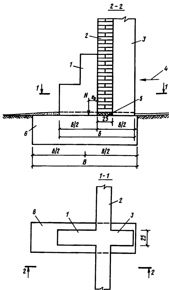
Черт. 59. Фундаменты под наружными стенами одноэтажных складских зданий для сыпучих материалов
