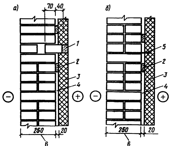
Черт. 31. Облегченная кладка типа В
