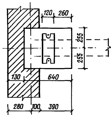
Черт. 9. Схема узла опирания балки на стену под опорной плитой в направлении оси балки
