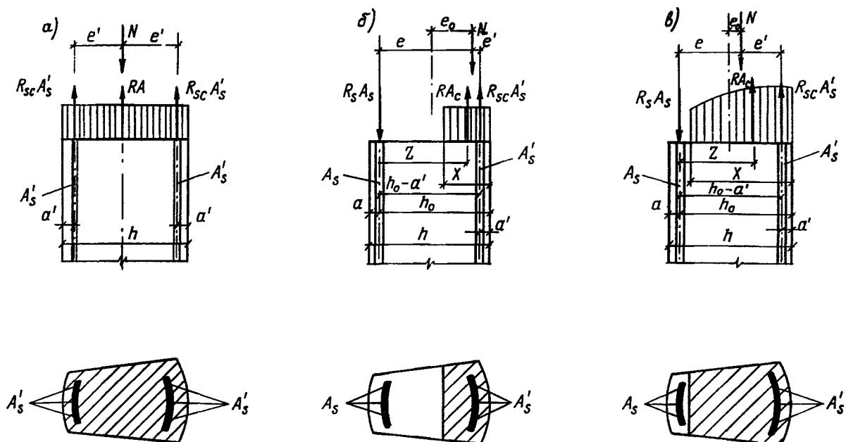
Черт. 13. Внецентренное сжатие армированной кладки
