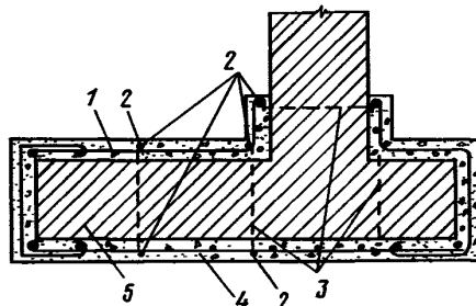
Черт. 16. Схема усиления стены железобетонной обоймой 1 – металлическая сетка; 2 – дополнительные стержни, расположенные сверх сетки; 3 – хомуты (связи); 4 – бетон обоймы; 5 – кладка стены
