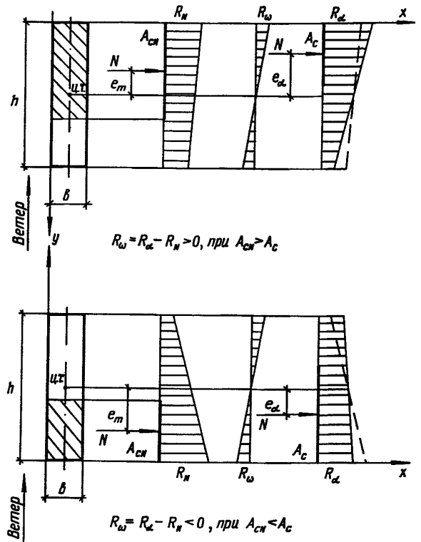
Черт. 7. Определение напряжений от действия ветровой и нормальной нагрузок на горизонтальные сечения стен в уровне \alpha -го этажа
