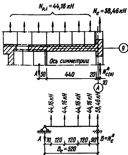
Черт. 13. Расчетная схема лестничной клетки
