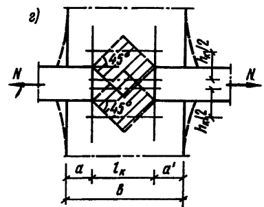
Черт. 3. Примеры построения зон влияния продольной силы N в кладке стен и перекрытий
