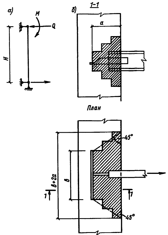
Черт. 55. Расчет анкера
