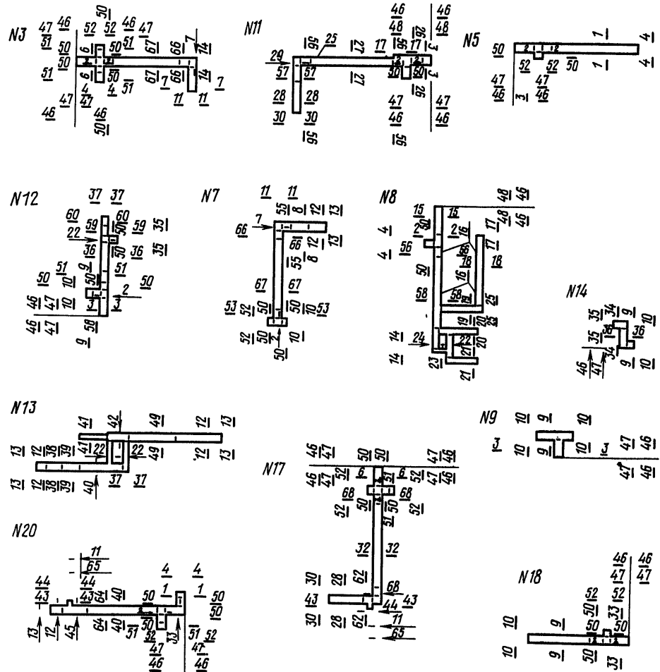
Черт. 10. Горизонтальные сечения всех стен здания (элементов)
