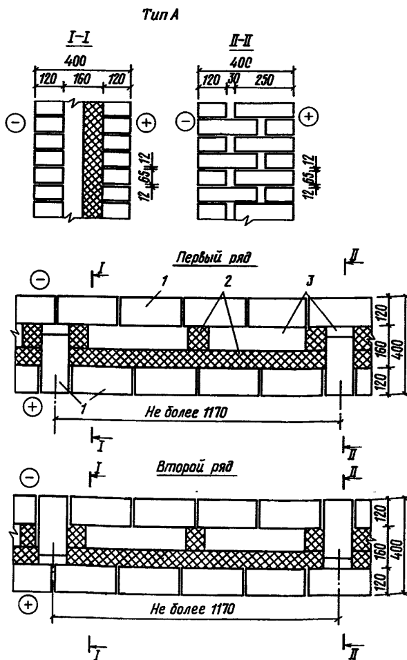
Черт. 29. Облегченная кладка типа А
