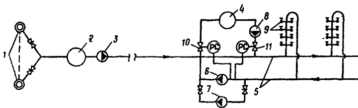
Рис. 2. Открытая однотрубная геотермальная система горячего водоснабжения с двухтрубной распределительной сетью
