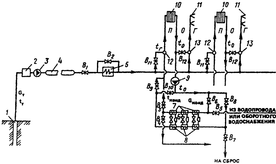
Рис. 13. Система децентрализованного теплохладоснабжения с тепловыми насосами
