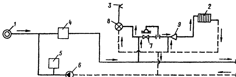
Рис. 10. Принципиальная схема бесливной системы геотермального теплоснабжения
