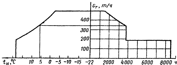
Рис. 2. График продолжительности расхода геотермального теплоносителя
