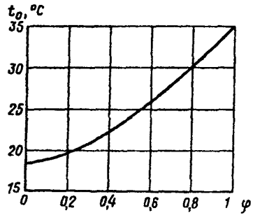
Рис. 2. График температуры обратной воды при количественном регулировании отопительной нагрузки ( t''_r = 80 °C, t''_o = 35 °C, t_b = 18 °C)
