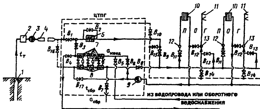
Рис. 12. Система централизованного теплохладоснабжения с тепловыми насосами
