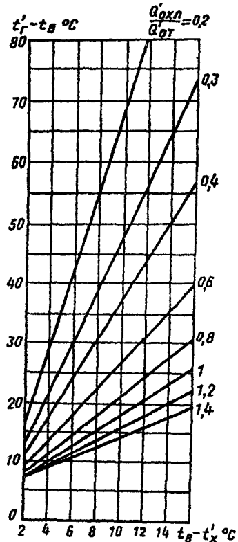
Рис. 7. Зависимость температуры теплоносителя от температуры хладоносителя и соотношения холодо- и тепловых нагрузок для радиационных систем отопления
