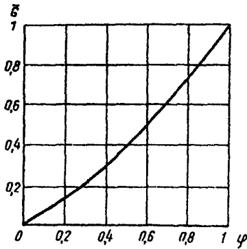
Рис. 1. График расхода теплоносителя при количественном регулировании отопительной нагрузки ( t''_r = 80 °C, t''_o = 35 °C, t_b = 18 °C)
