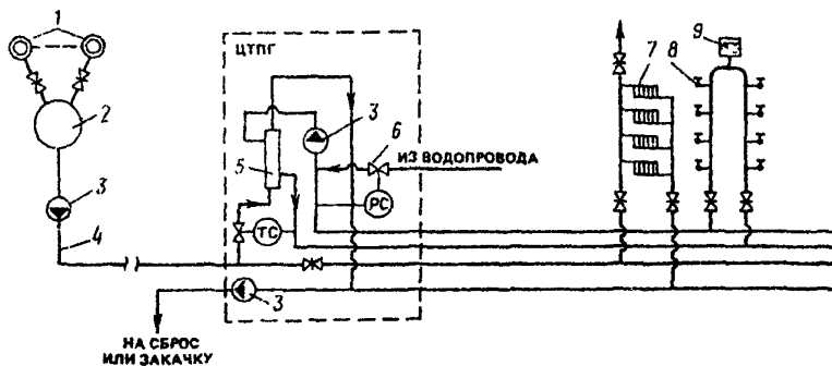
Рис. 6. Закрытая однотрубная геотермальная система теплоснабжения с зависимым присоединением отопления (распределительная сеть четырехтрубная)
