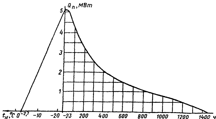
Рис. 1. График продолжительности тепловой нагрузки пикового источника теплоты
