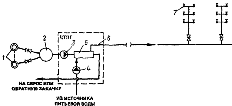
Рис. 4. Однотрубная закрытая геотермальная система горячего водоснабжения с источником питьевой воды, расположенным на термоводозаборе 1 — геотермальные скважины термоводозабора; 2 — сборный бак-аккумулятор геотермальной воды; 3 — сетевой насос геотермальной воды; 4 — сетевой насос питьевой воды; 5 — сетевой теплообменник; 6 — однотрубная транзитная теплотрасса; 7 — водоразборный кран
