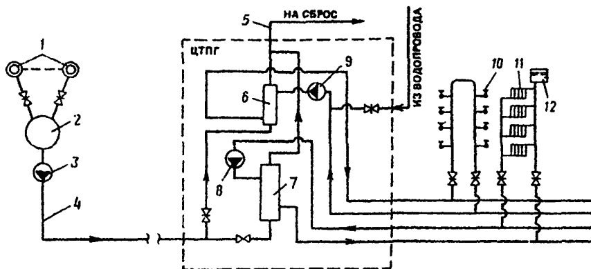
Рис. 7. Закрытая геотермальная система теплоснабжения с независимым присоединением отопления
