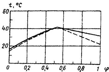
Рис. 3. Температура сбросной геотермальной воды — — — — комплексная система с пиковой котельной; - - - - - то же, с ТНУ
