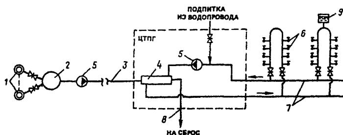
Рис. 5. Однотрубная закрытая геотермальная система горячего водоснабжения
