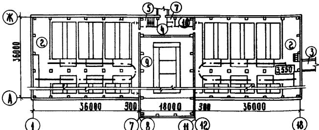
ПЛАН НА ОТМ. 3.550 и 3.600
