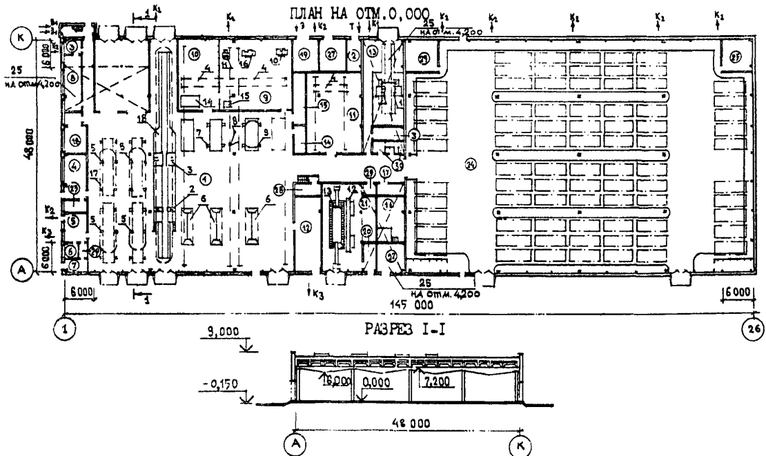
ЭКСПЛИКАЦИЯ ПОМЕЩЕНИЙ
