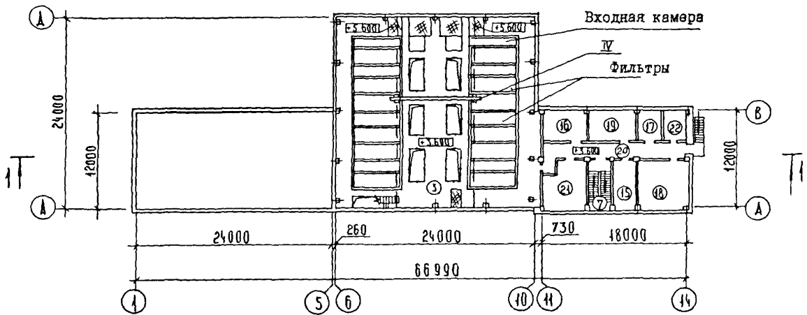
ПЛАН НА ОТМ. 3.600
