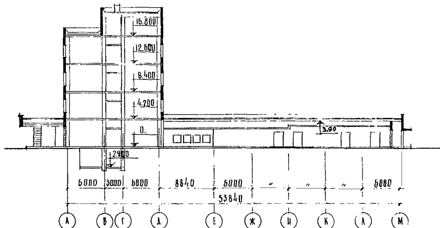
РАЗРЕЗ 2-2
