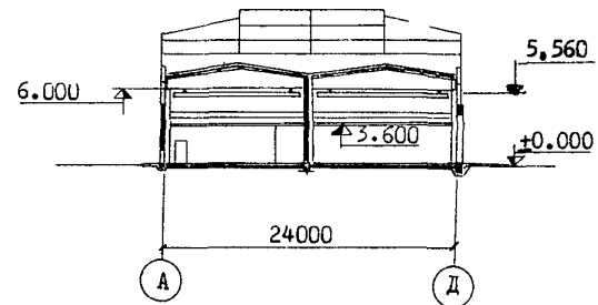
РАЗРЕЗ III - III
