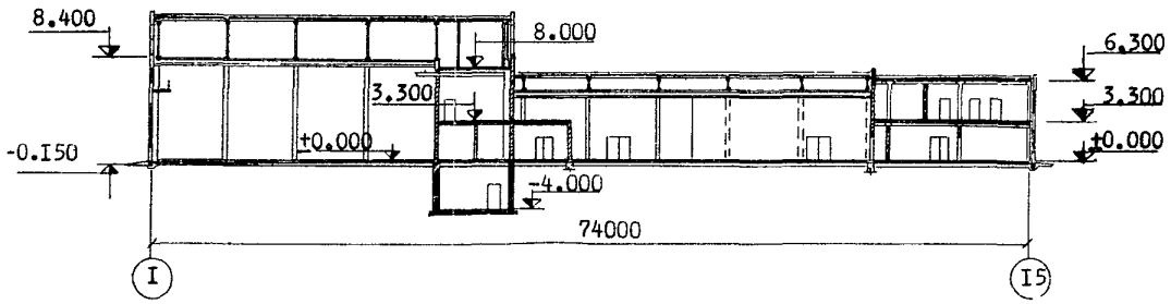
РАЗРЕЗ I - I
