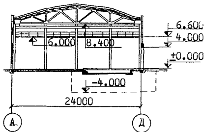
РАЗРЕЗ II - II
