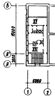
ПЛАН НА ОТМ. 3,30
