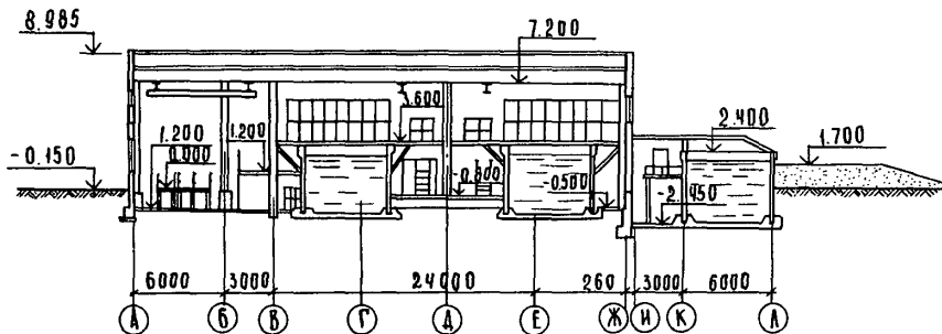
РАЗРЕЗ I-I
