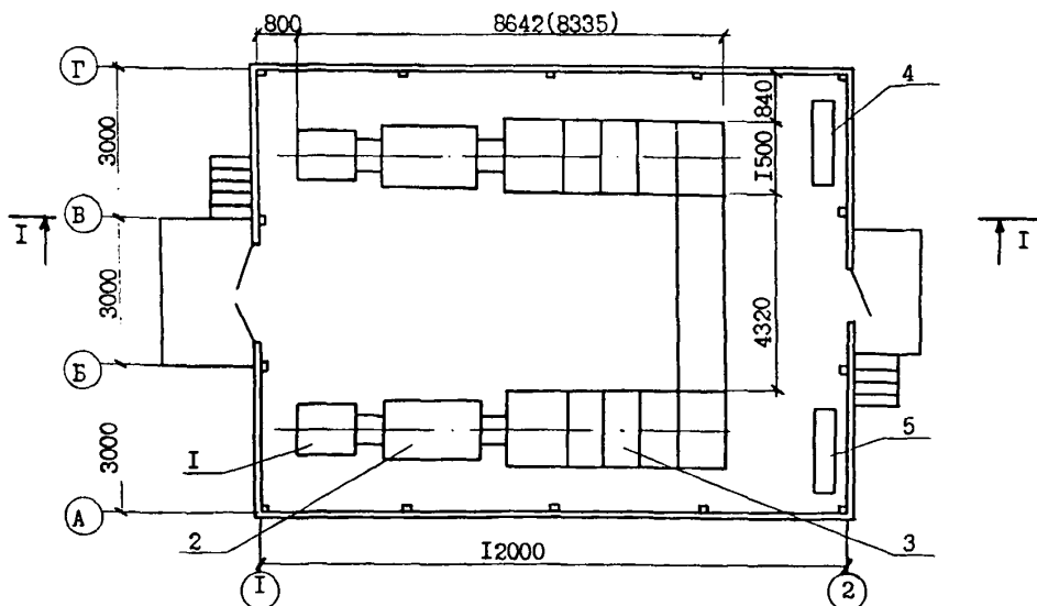
ЭКСПЛИКАЦИЯ ОБОРУДОВАНИЯ
