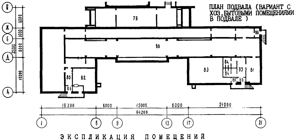
ЭКСПЛИКАЦИЯ ПОМЕЩЕНИЙ
