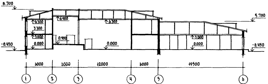
РАЗРЕЗ I-I
