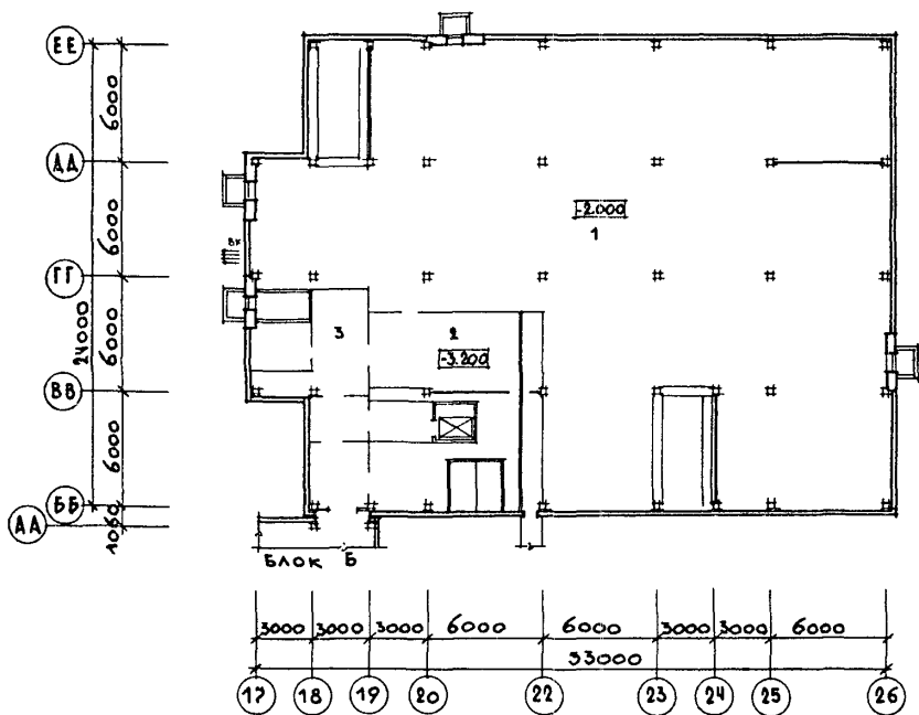
БЛОК В. ПЛАН ТЕХПОДПОЛЯ И ПОДВАЛА
