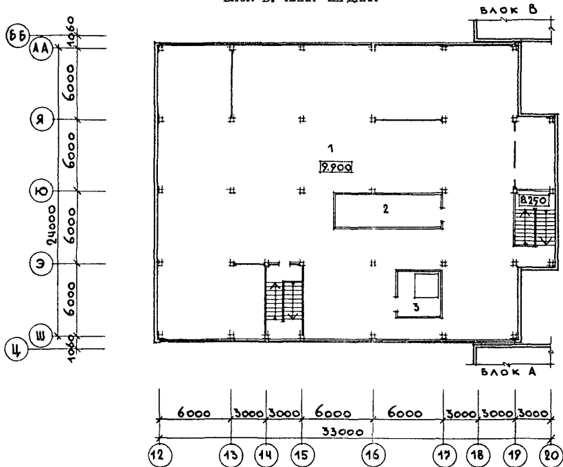
БЛОК Б. ПЛАН ЧЕРДАКА
