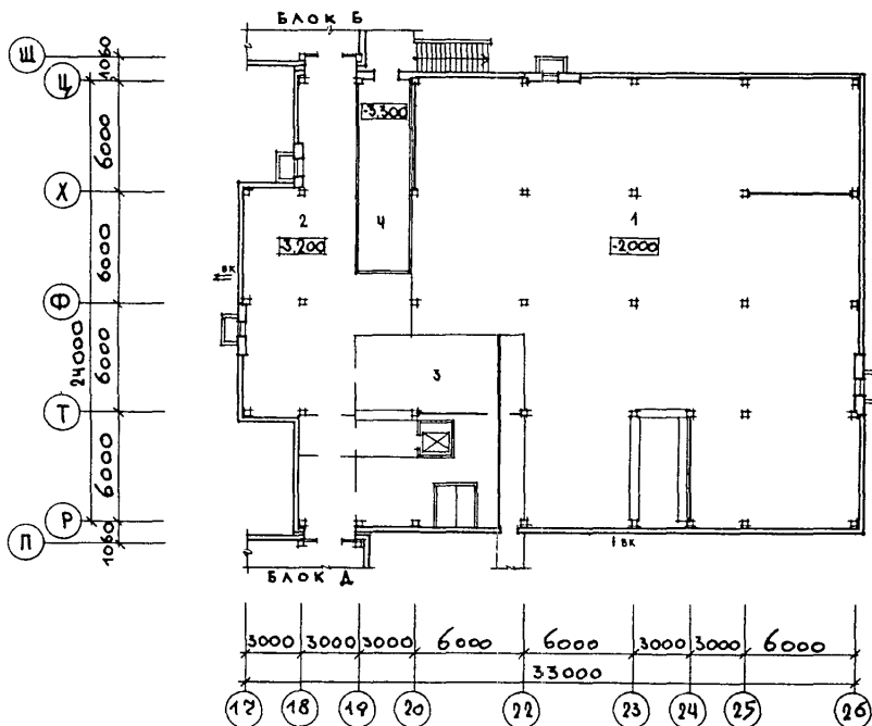
БЛОК А. ПЛАН ТЕХПОДПОЛЯ И ПОДВАЛА
