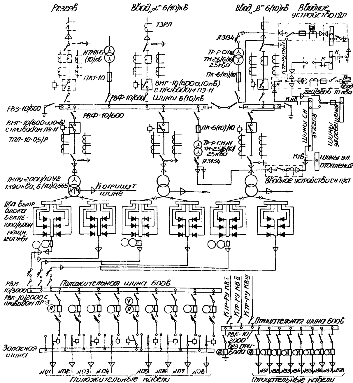
Схема электрических соединений
